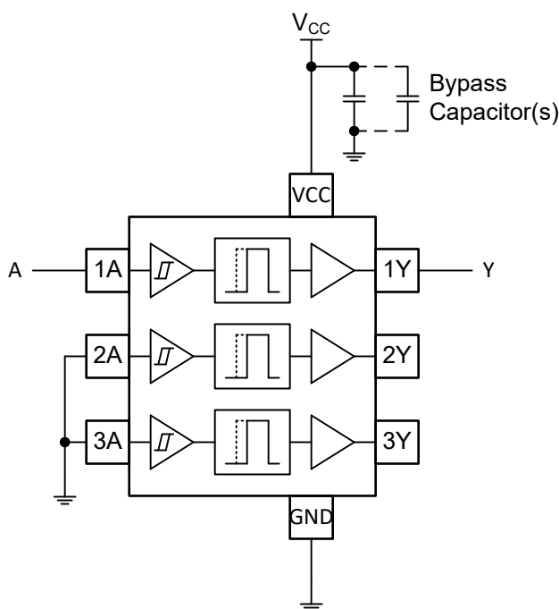
图 8-1. 使用 TDEL3G511-Q1 的上升沿延迟原理图
