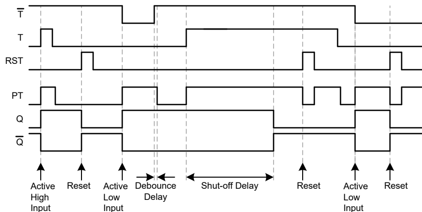
图 5-1. 时序图
