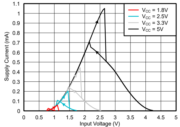
图 5-5. 输入电压与电源电流间的关系
