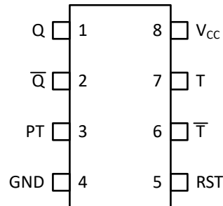
引脚排列图
