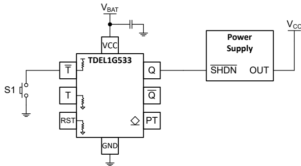
功能方框图
