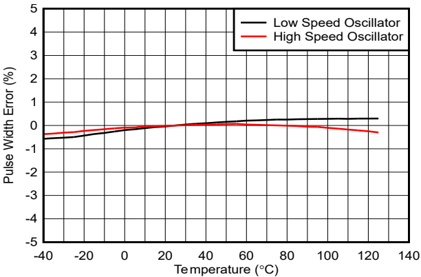
图 5-2. 脉宽误差与温度之间的关系
