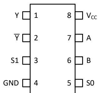
图 4-1. TDEL1G522-Q1 DRL 封装 ( 顶视图 )
