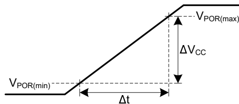
图 7-2. 已知上电状态的电源 ( V_{\text{CC}} ) 斜坡特性
