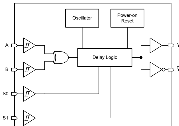
功能方框图
