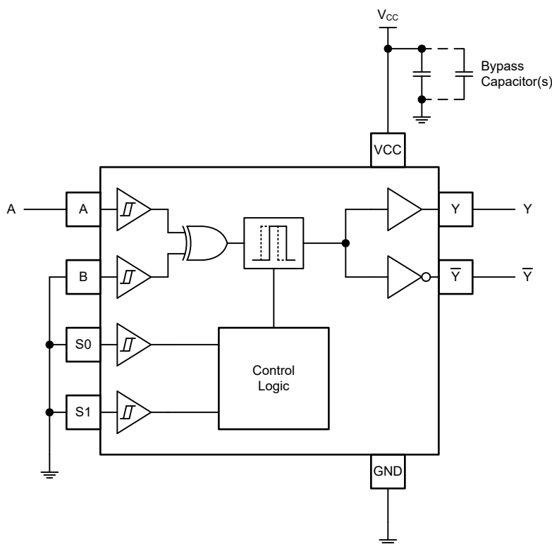
图 8-1. 使用 TDEL1G522-Q1 的延迟原理图
