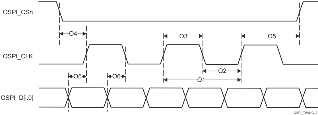
图 6-104. OSPI/1 开关特性 - PHY DDR 数据训练
