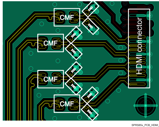
图 7-43. HDMI Placement Diagram
