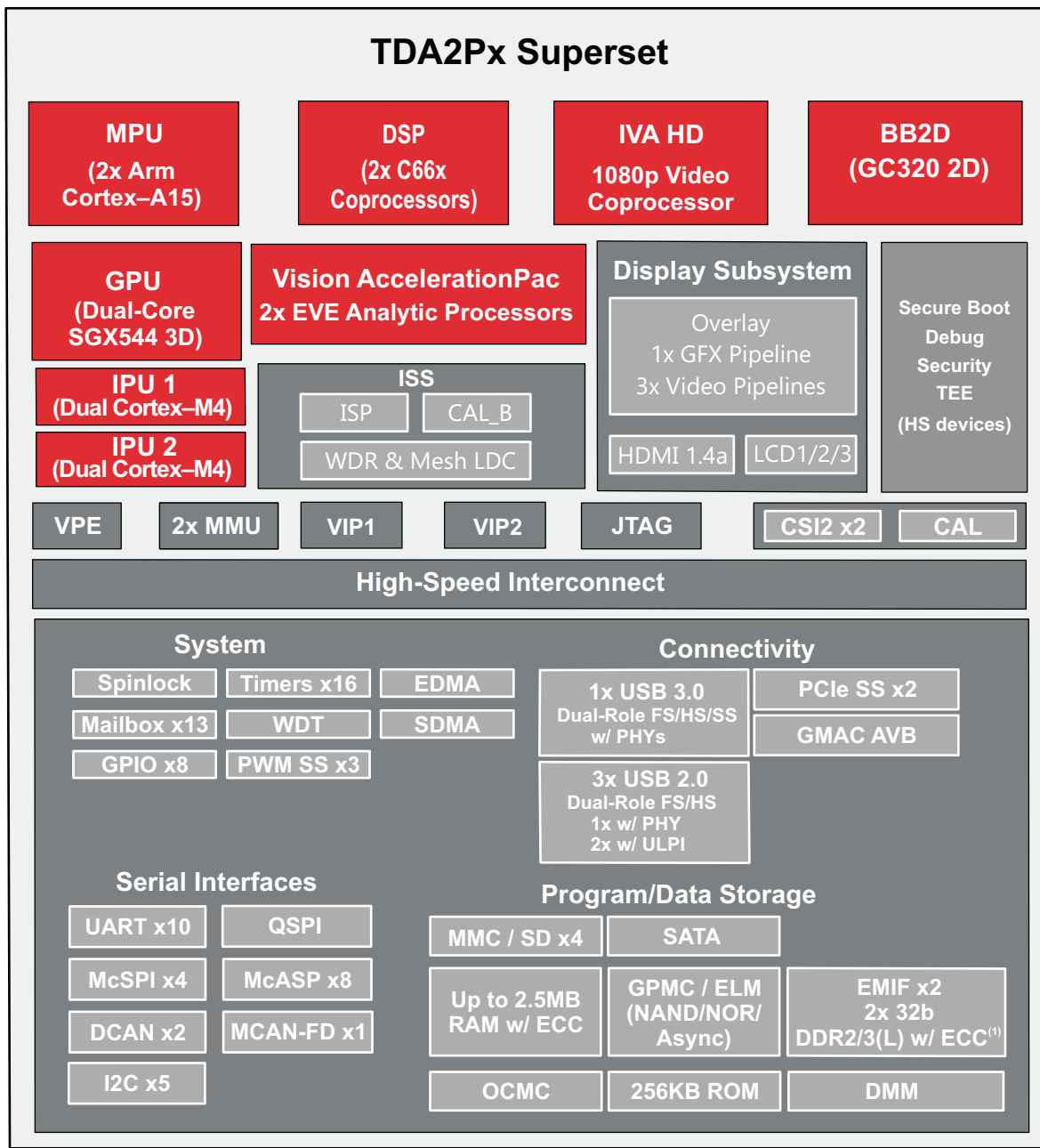
图 1-1. TDA2Px 方框图
