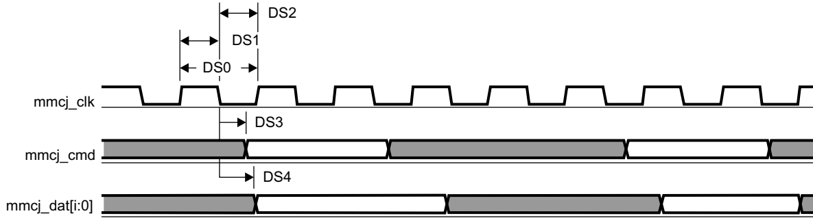
图 5-92. MMC/SD/SDIOj in - Default Speed - Transmitter Mode
