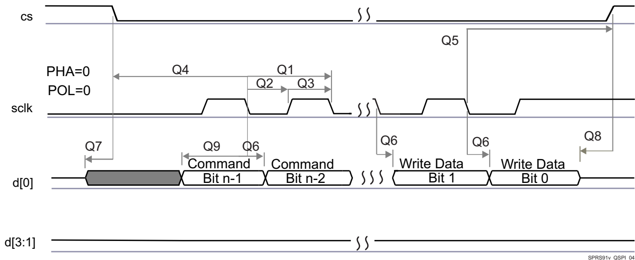
图 5-49. QSPI Write (Clock Mode 0)
