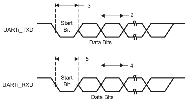
图 5-41. UART Timing
