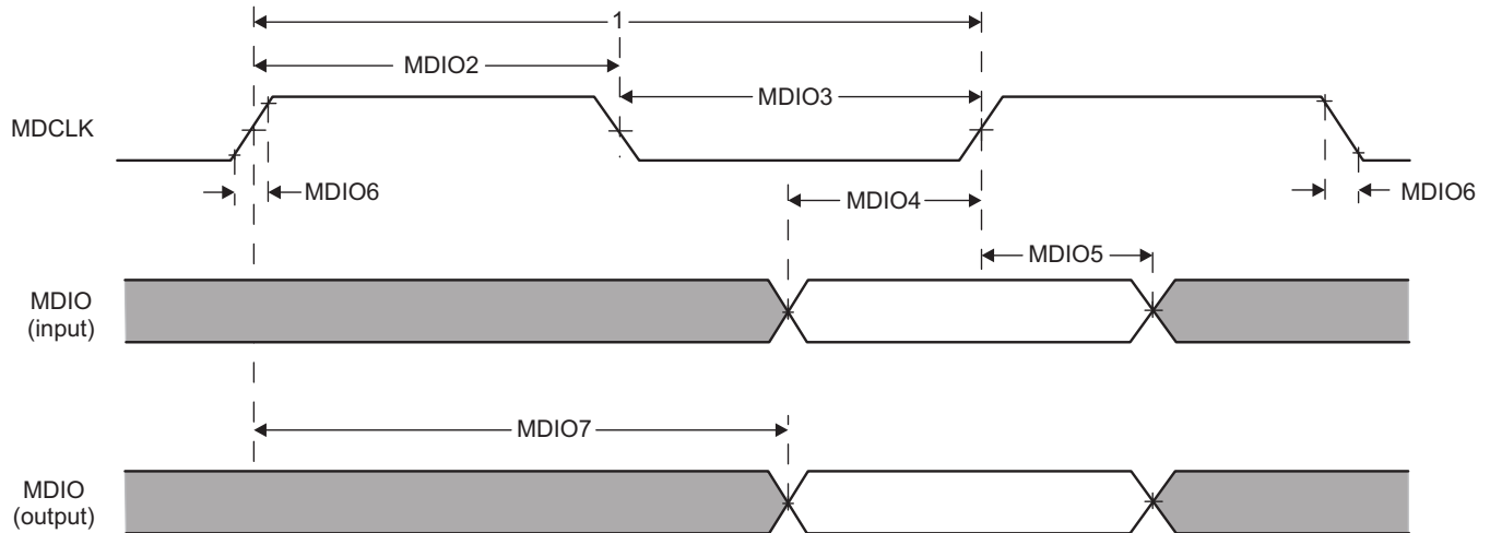
图 5-65. GMAC MDIO diagrams
