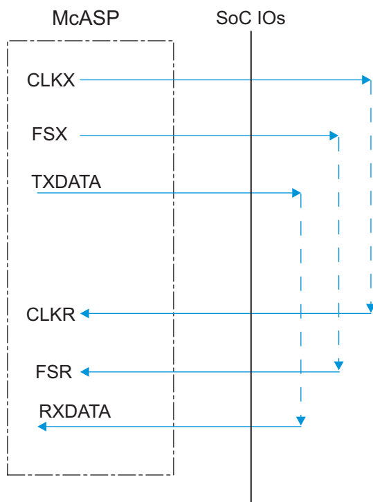
图 5-52. McASP1-8 COIFOI – ASYNC Mode
