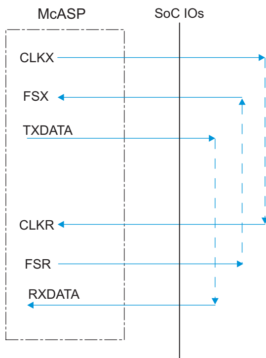
图 5-53. McASP1-8 COIFIO – ASYNC Mode
