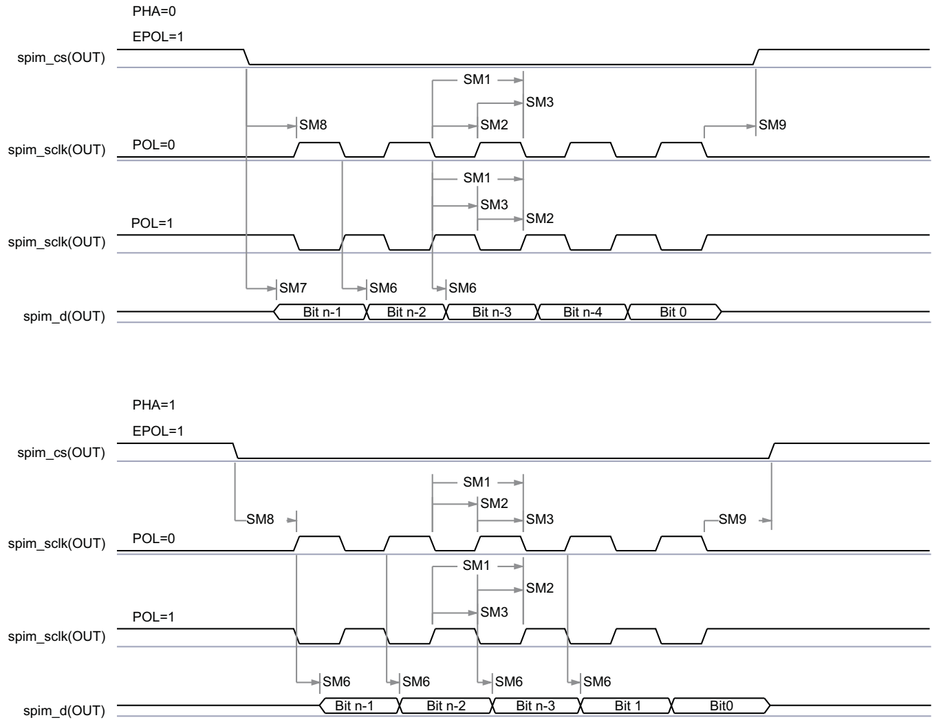
图 5-42. McSPI - Master Mode Transmit
