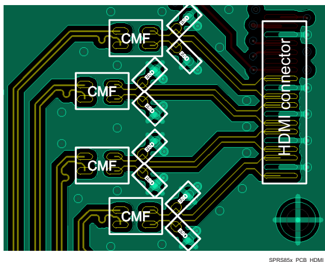
图 7-34. HDMI Placement Diagram
