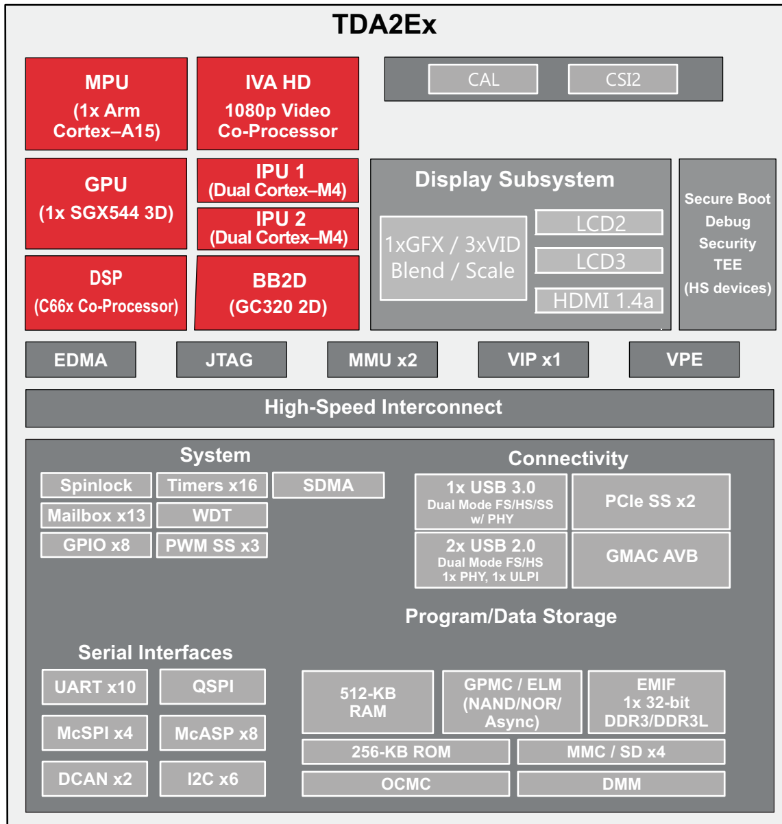
图 1-1. TDA2Ex 框图
