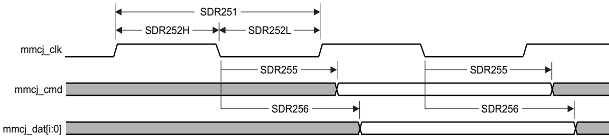
图 5-98. MMC/SD/SDIOj in - SDR25 - Transmitter Mode
