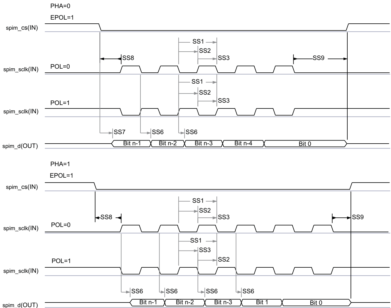
图 5-44. McSPI - Slave Mode Transmit
