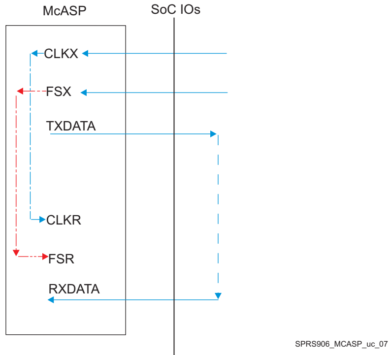
图 5-58. McASP1-8 CI-FI – SYNC Mode
