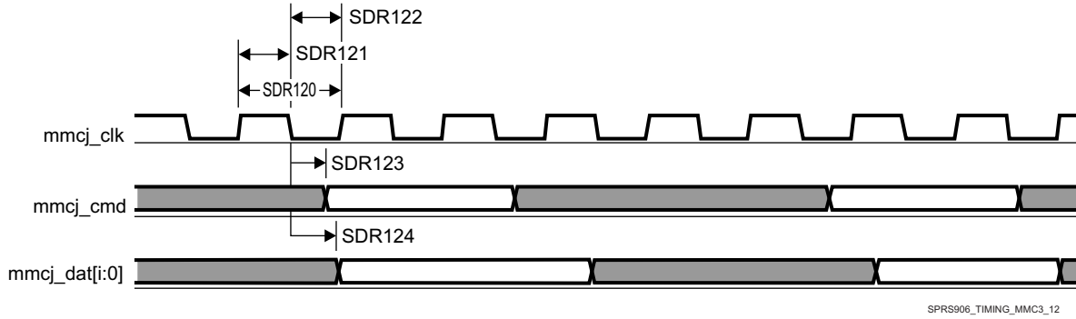
图 5-96. MMC/SD/SDIOj in - SDR12 - Transmitter Mode
