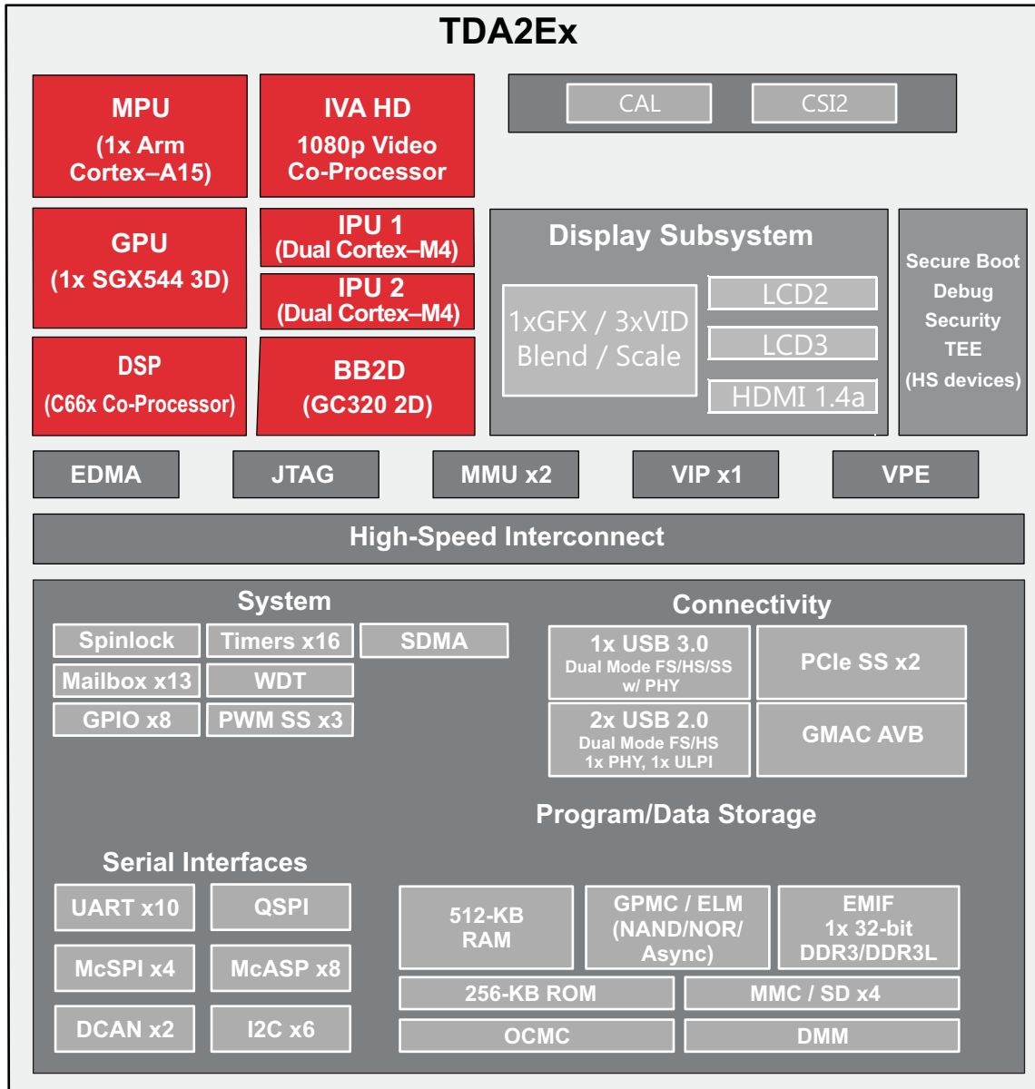
图 6-1. TDA2Ex Block Diagram
