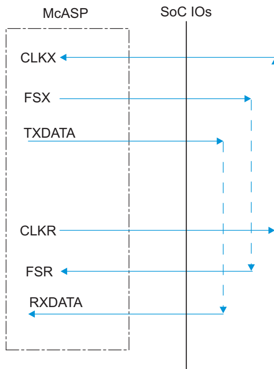
图 5-55. McASP1-8 CIOFOI – ASYNC Mode
