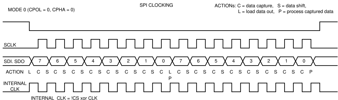
图 33. SPI Clocking
