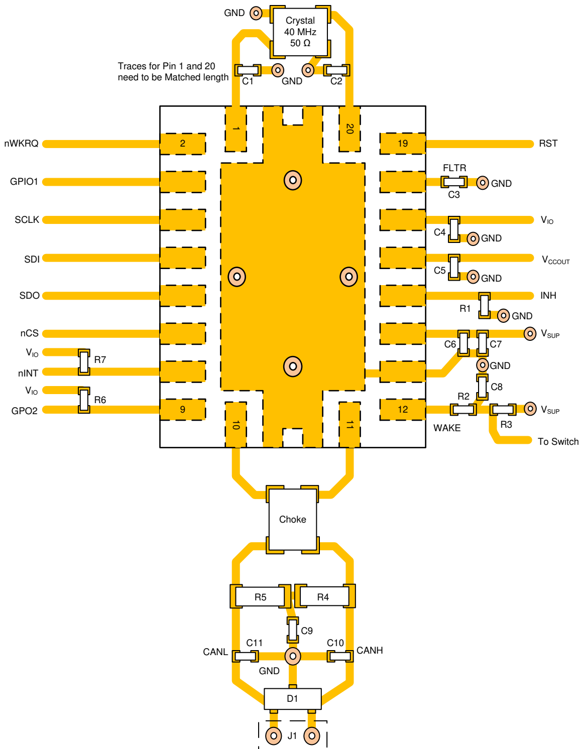
图 113. Example Layout
