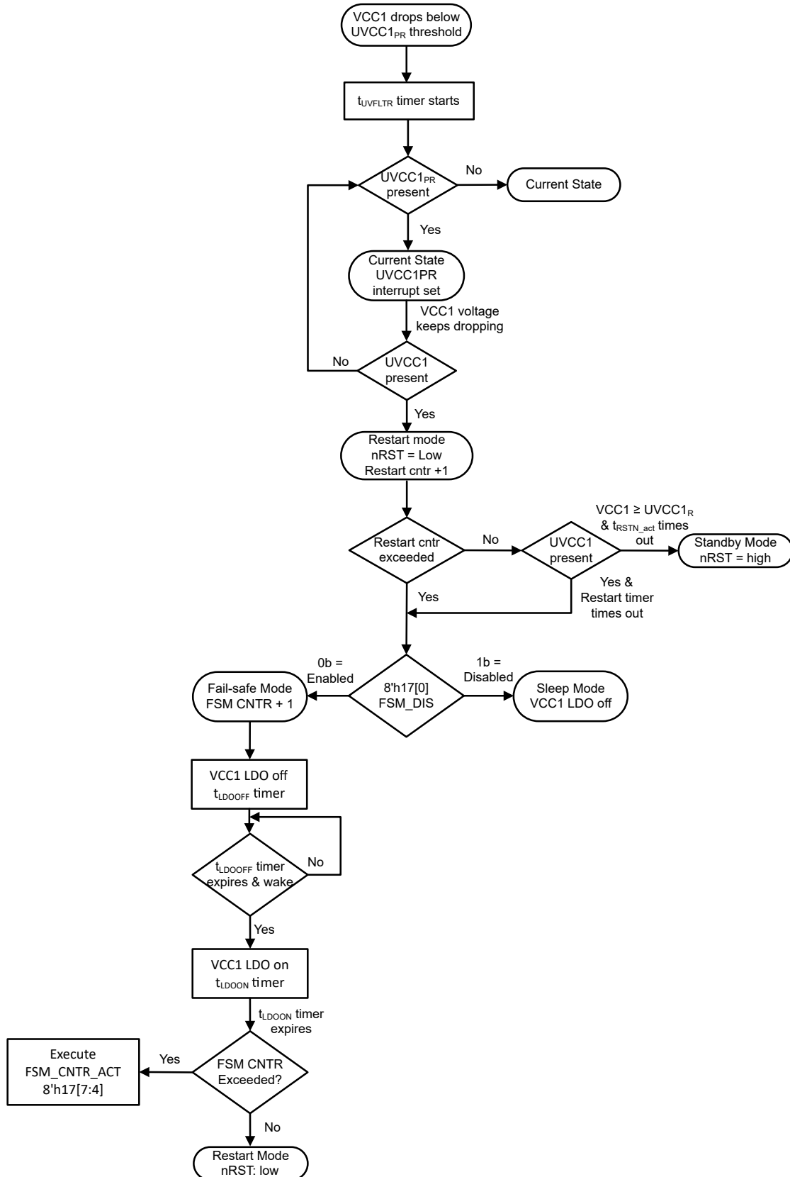
图 8-47. UVCC1 状态图
