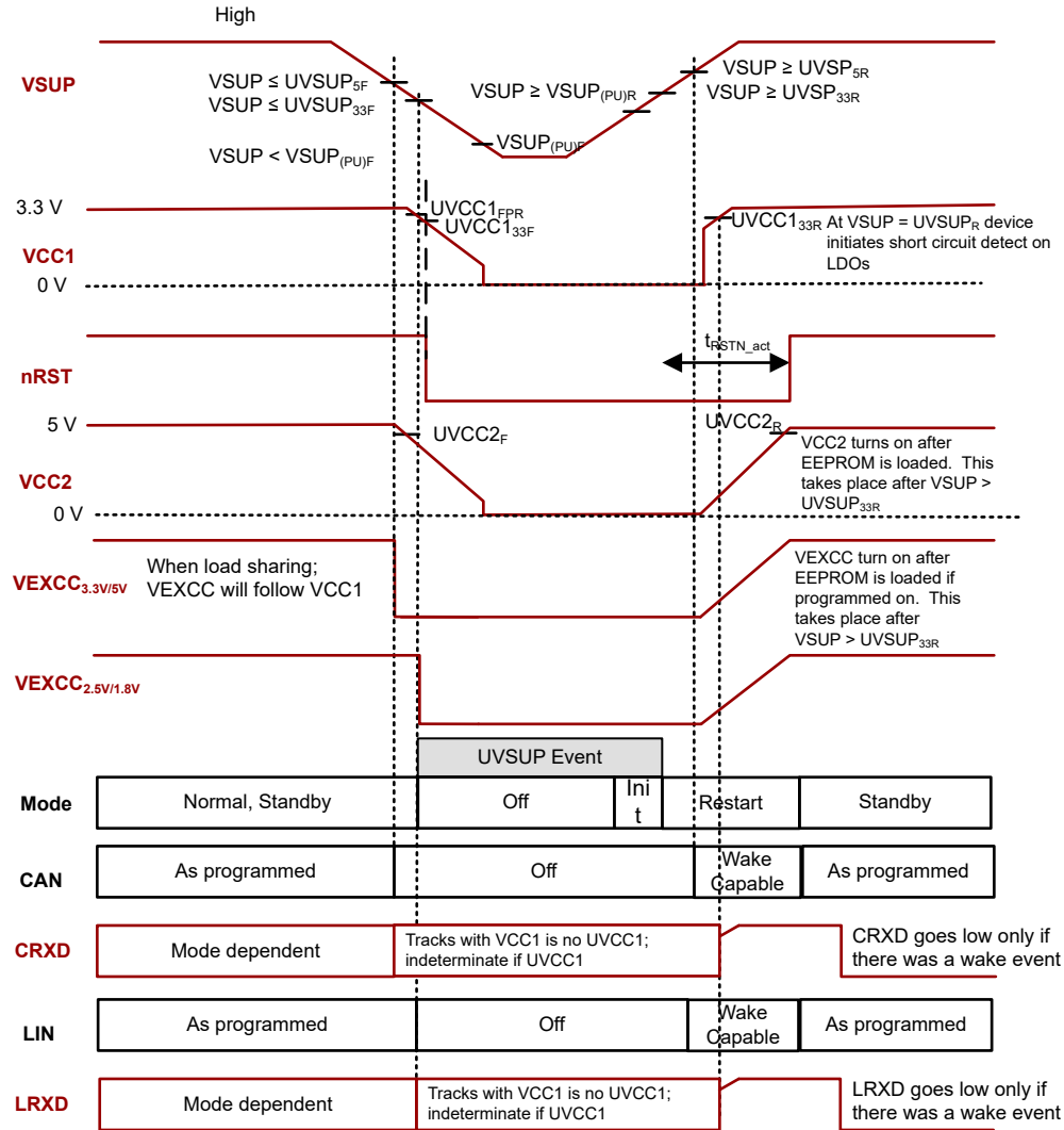
图 10-11. VCC1 = 3.3V 时，欠压低于 VSUP_{(PU)F} 欠压
