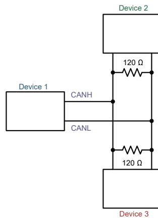
图 8-66. 三节点示例
