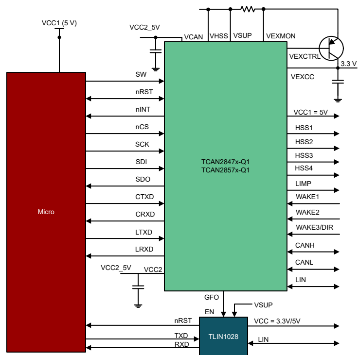
图 10-5. 使用 LIN SBC 进行通道扩展
