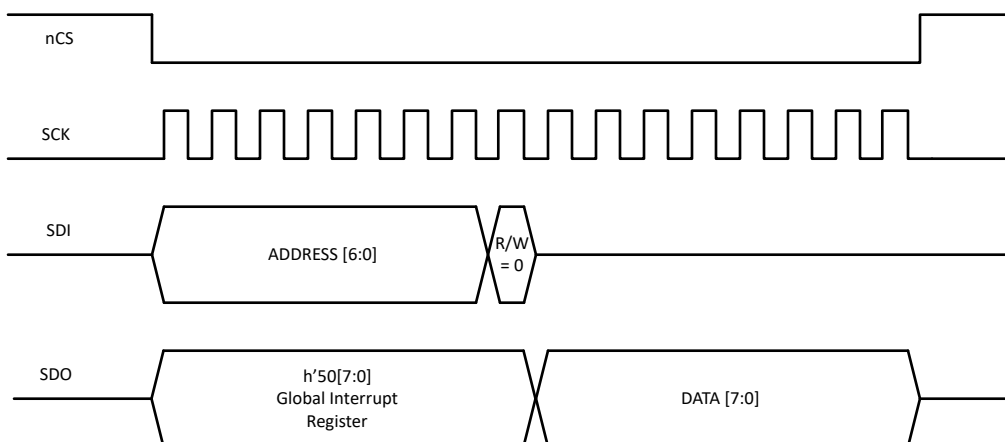
图 8-73. SPI 读取
