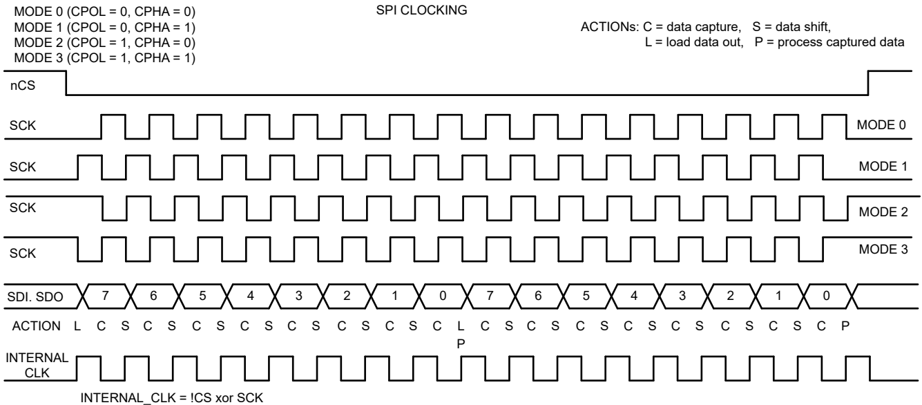
图 8-78. SPI 时钟
