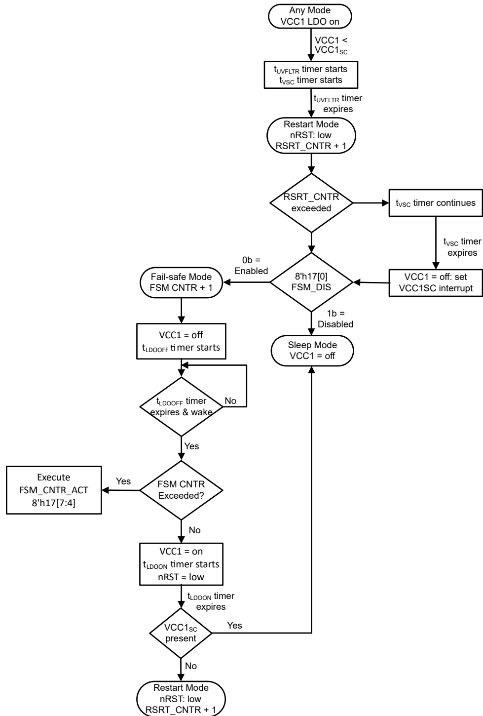
图 8-54. VCC1SC 状态图
