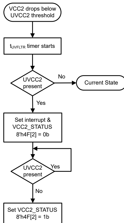
图 8-48. UVCC2 状态图
