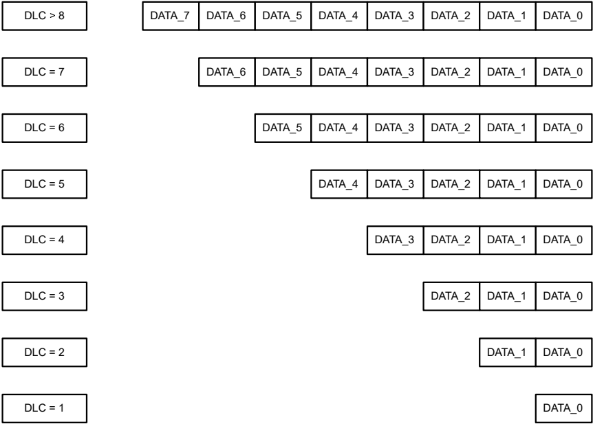
图 8-40. 不同 DLC 值的数据寄存器掩码值
