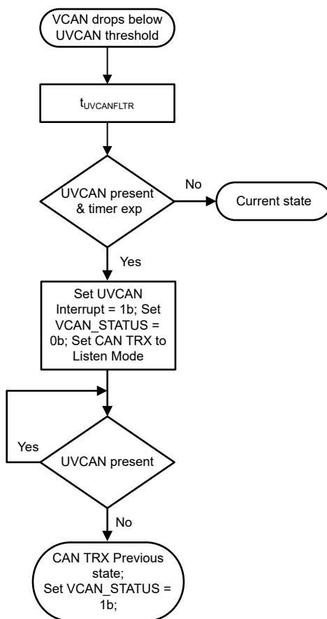
图 8-50. UVCAN 状态图
