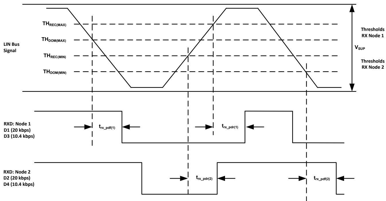
图 7-14. LIN 传播延迟
