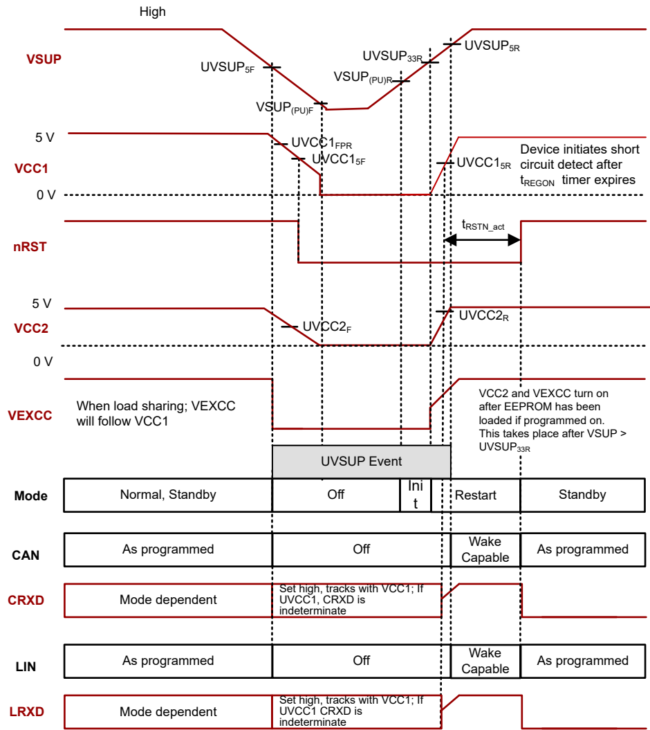
图 10-9. VCC1 = 5V 时，欠压低于 VSUP (PU)F 欠压
