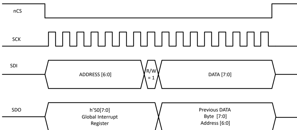
图 8-72. SPI 写入
