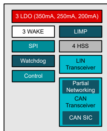
TCAN2847-Q1 示意图
