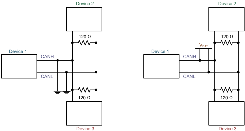
图 8-71. 短路故障 10 和 11 示例
