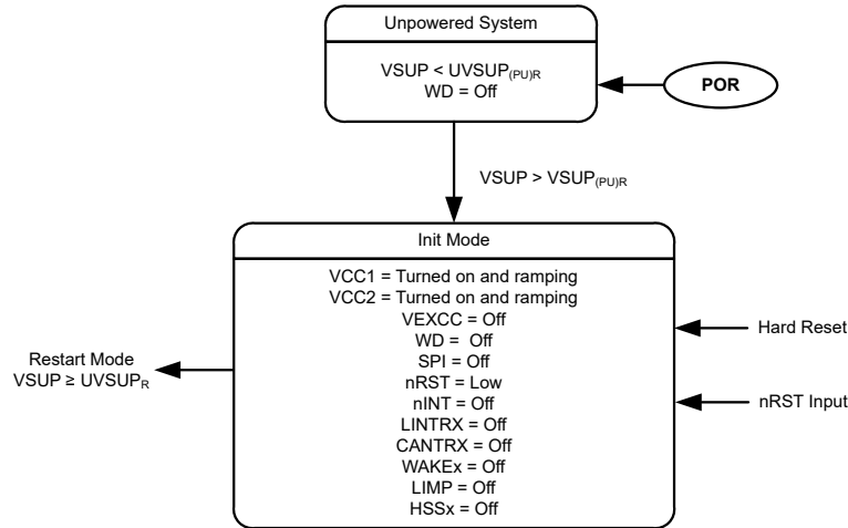
图 8-21. 初始化模式
