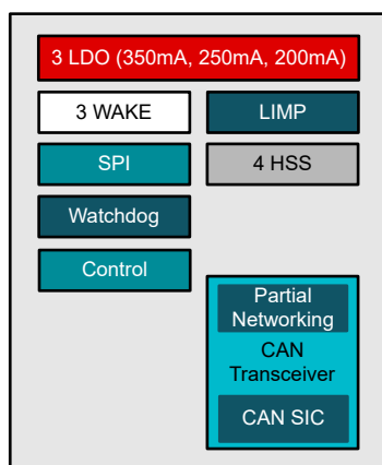
TCAN2845-Q1 示意图
