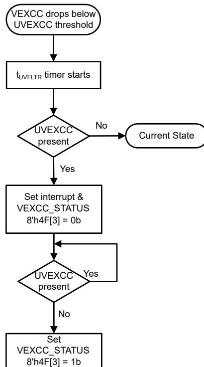
图 8-49. UVEXCC 状态图
