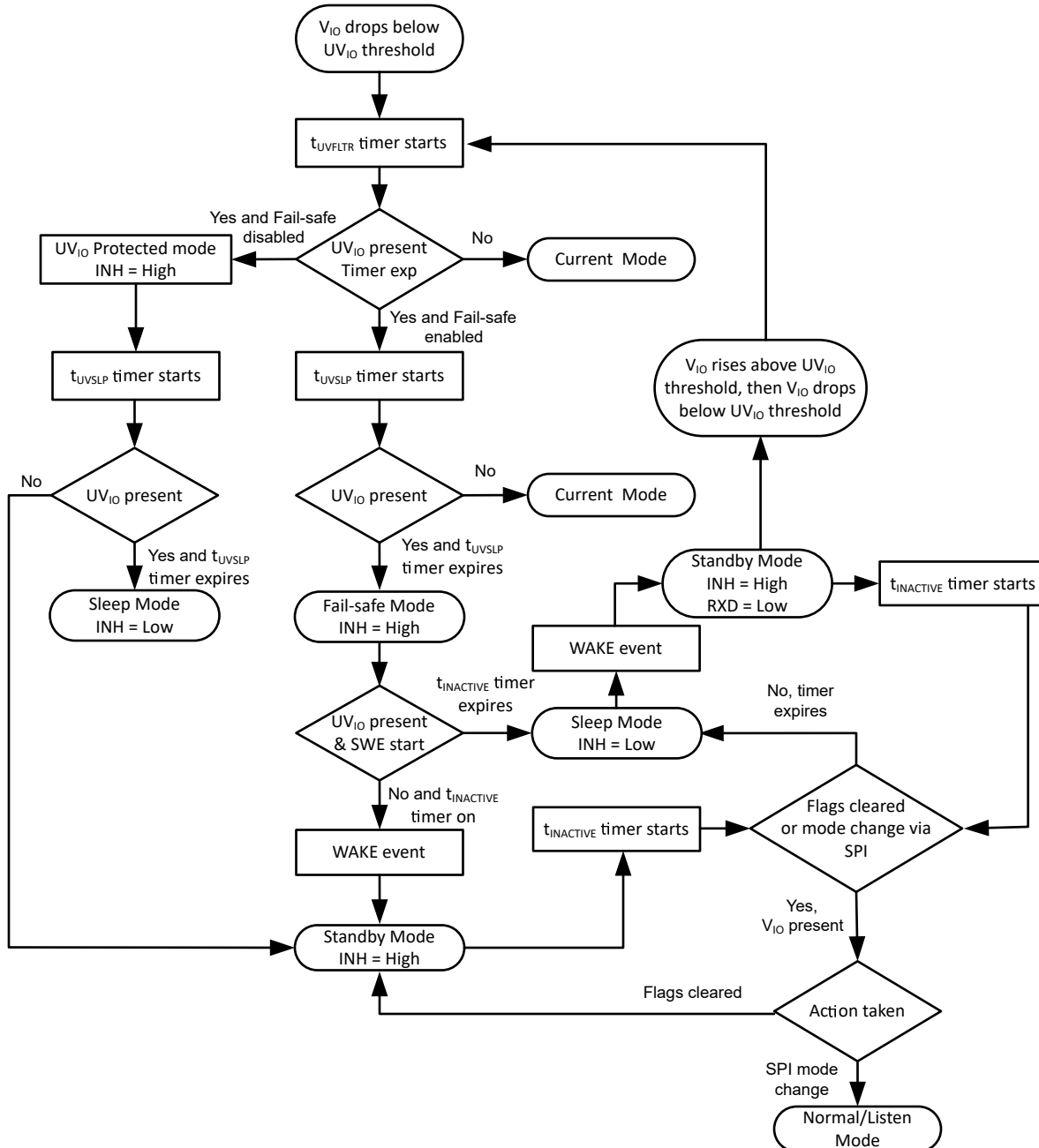
图 8-25. UV IO 状态图
