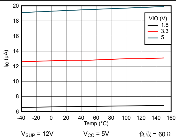
图 6-5. 正常模式显性 I_{IO} 与温度间的关系
