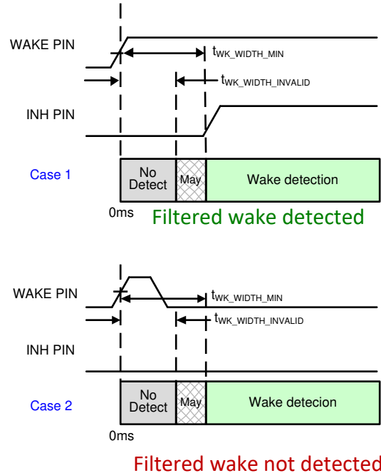
图 8-18. WAKE 引脚滤波行为
