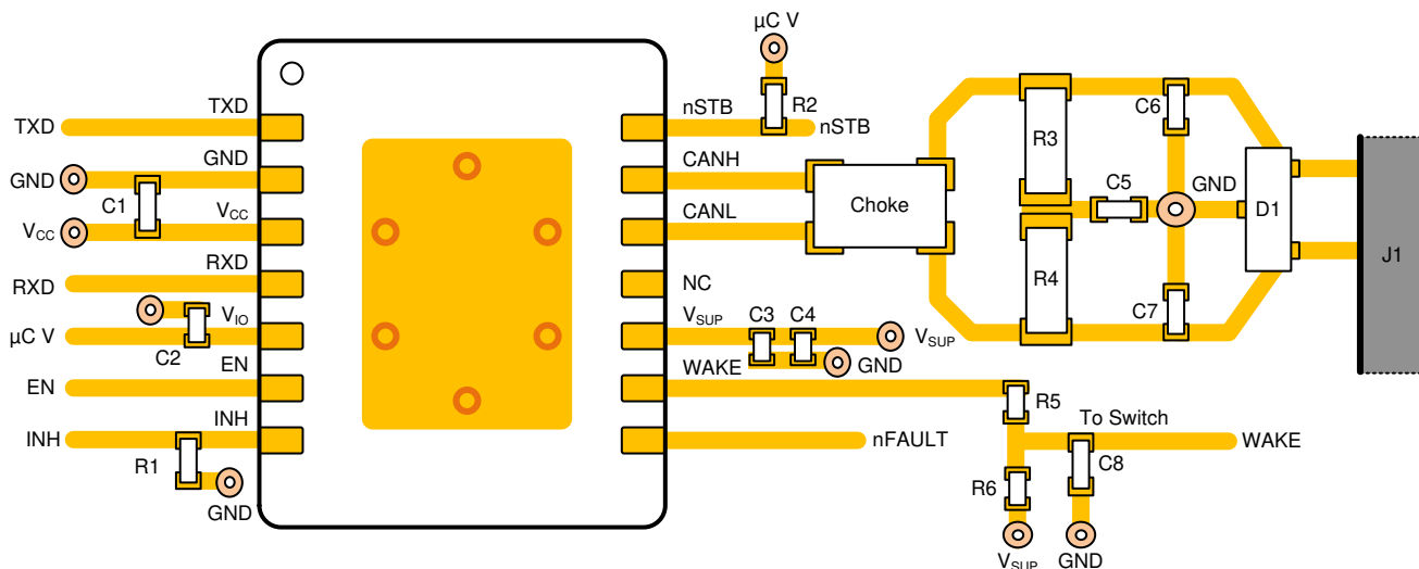
图 8-4. 示例布局
