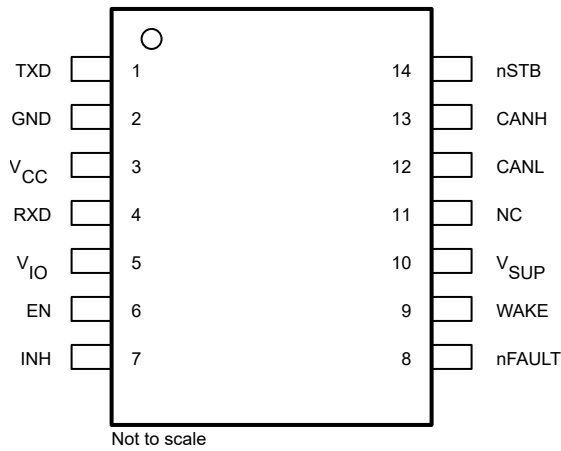
图 4-1. D 封装 14 引脚 (SOIC) (顶视图)
