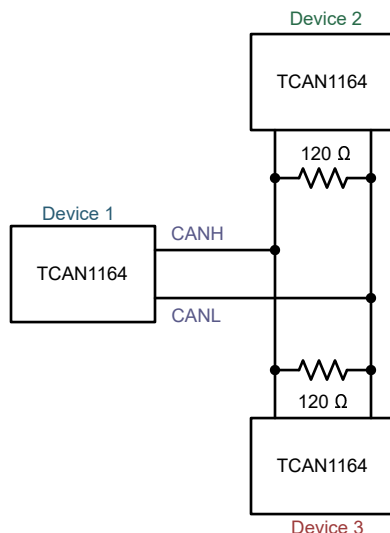
图 8-7. 三节点示例
