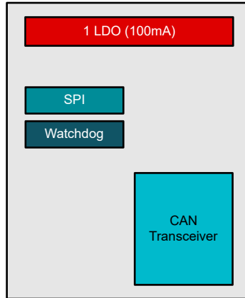
TCAN1164-Q1 示意图
