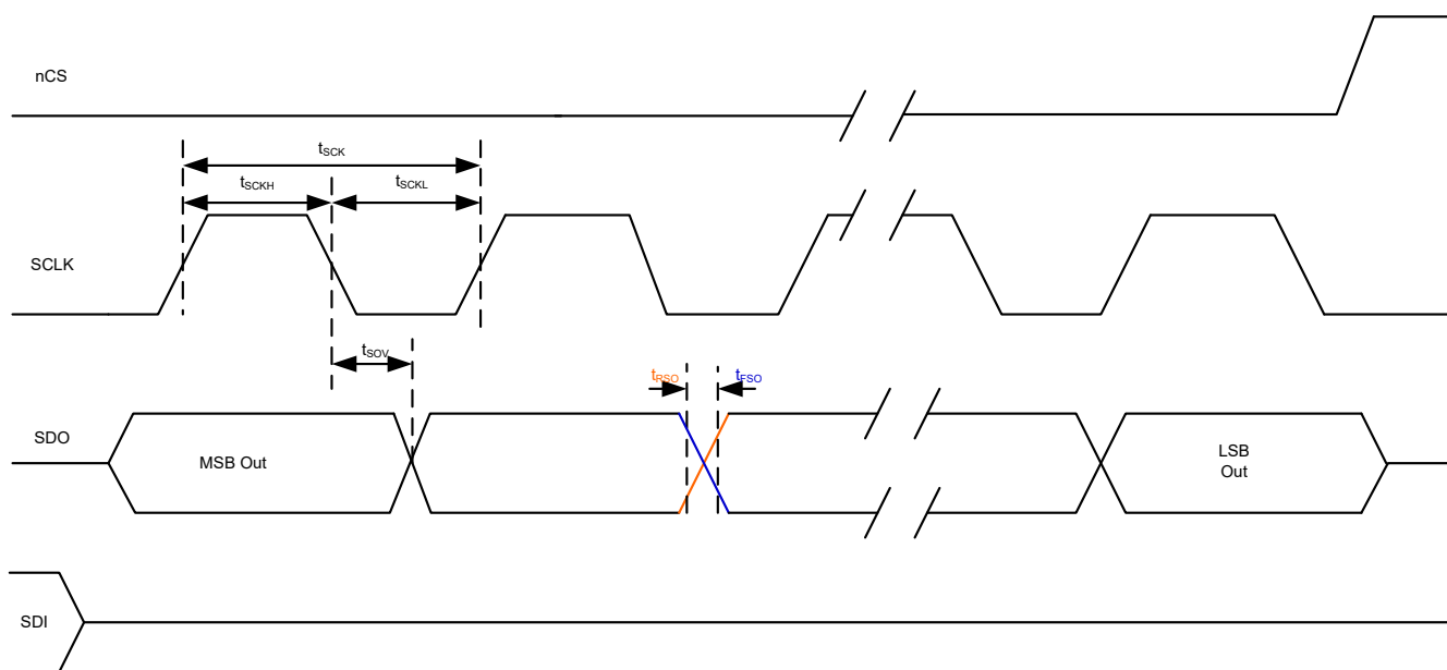
图 7-12. SPI AC 特征读取
