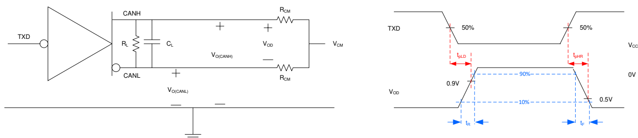
图 7-2. 驱动器测试电路与测量
