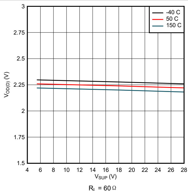
图 6-2. V_{\text{OD(DOM)}} 与 V_{\text{SUP}} 间的关系
