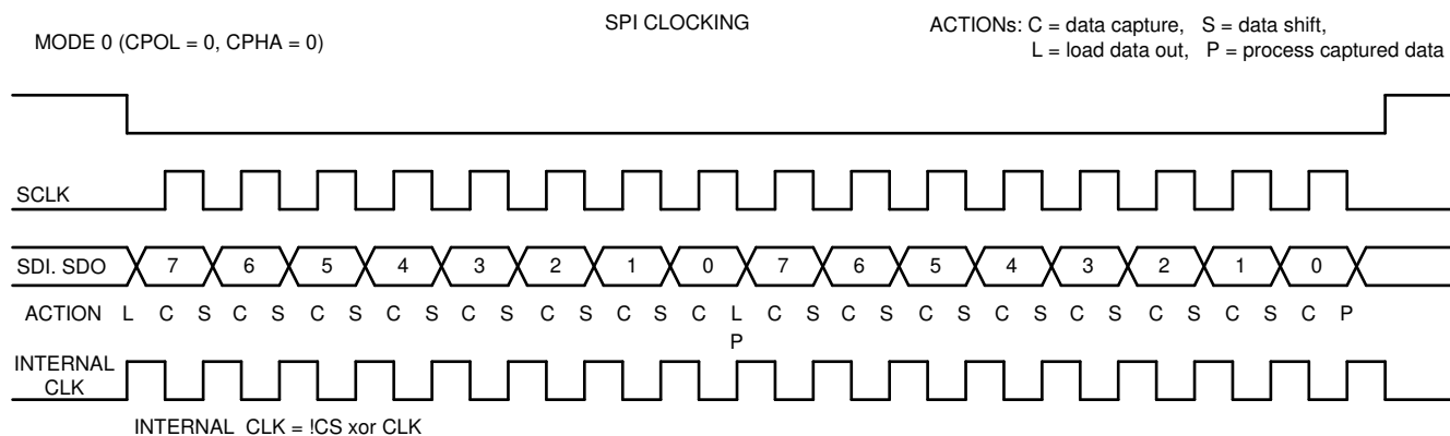
图 8-17. SPI 时钟
