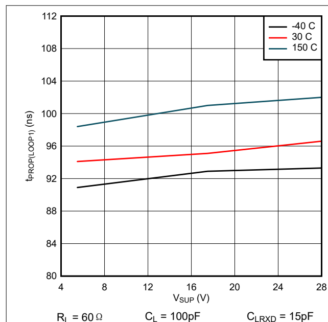
图 6-1. t_{\text{PROP(LOOP1)}} 与 V_{\text{SUP}} 间的关系
