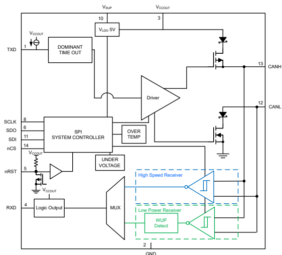
功能方框图
