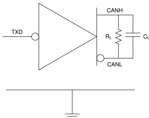
图 7-1. I_{SUP} 测试电路
