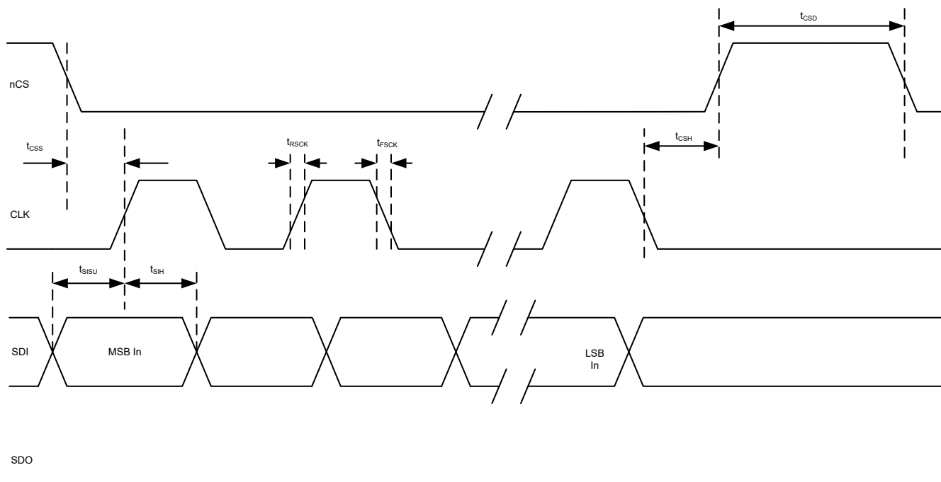
图 7-11. SPI AC 特征写入
