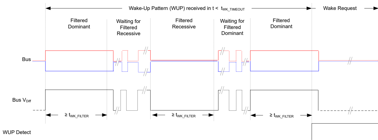
图 8-14. 唤醒模式 (WUP)
