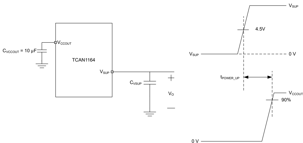
图 7-9. t_{POWER\_UP} 时序测量
