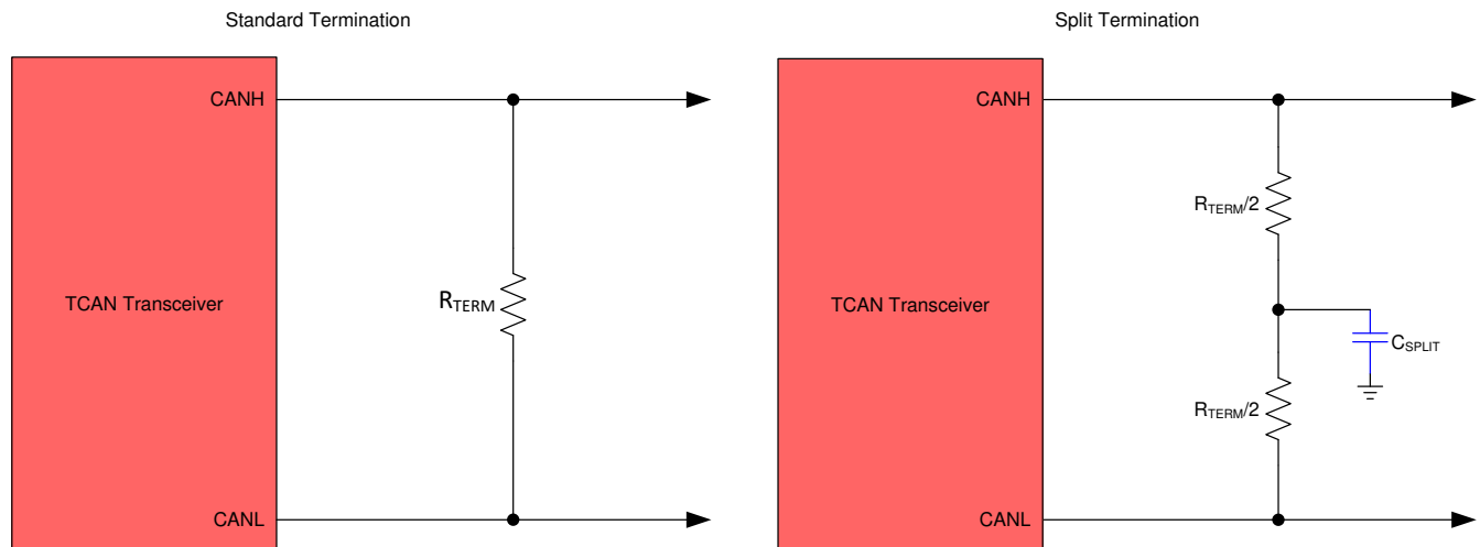
图 9-2. CAN 总线端接概念
