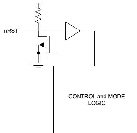
图 8-1. nRST 电路
