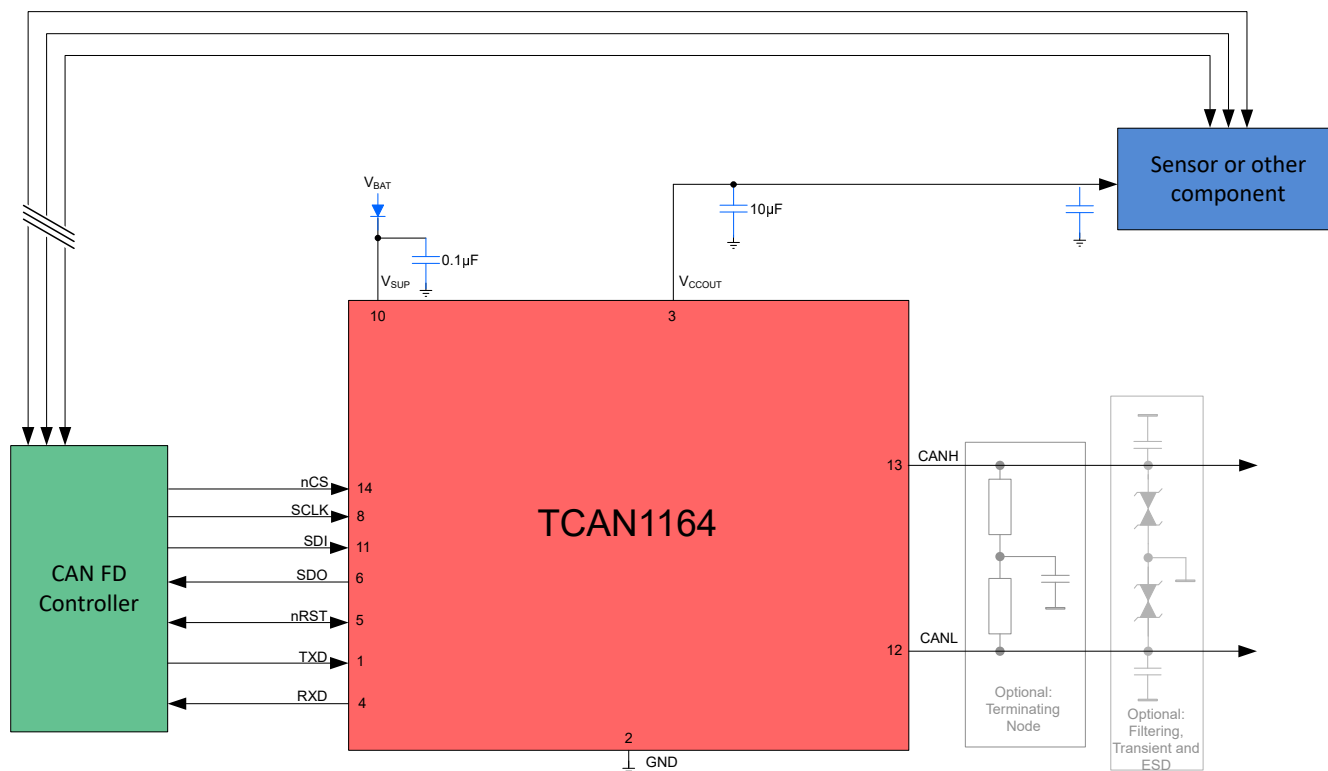
图 9-1. 典型应用
