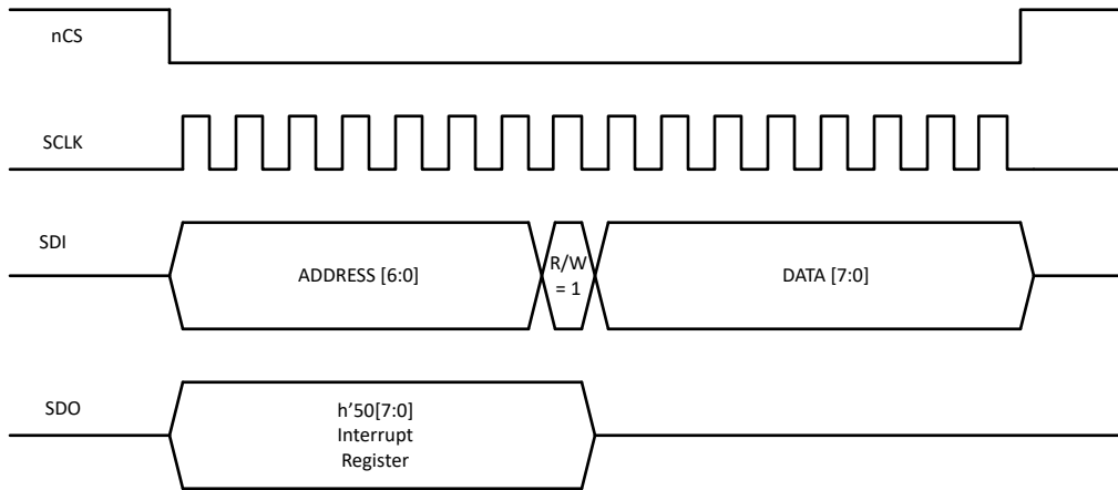
图 8-18. SPI 写入
