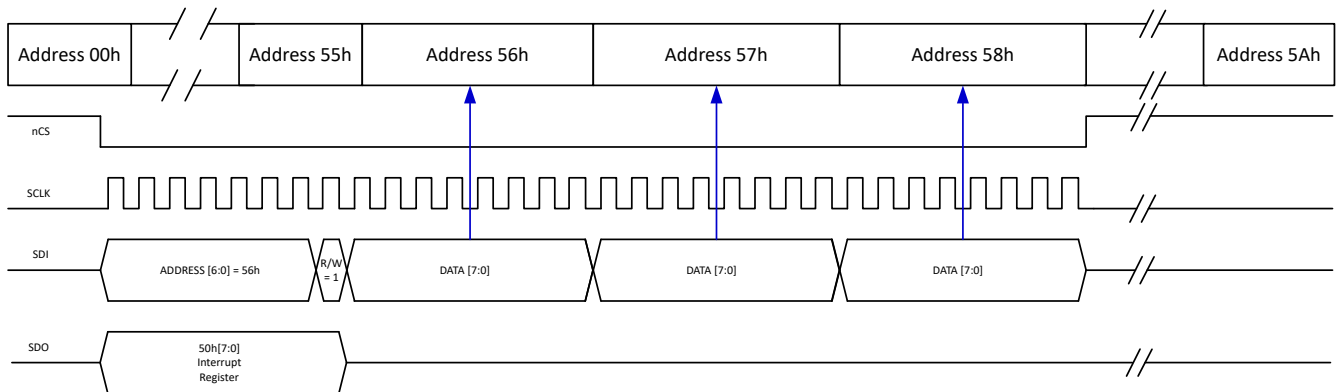
图 8-19. 32 位 SPI 突发写入
