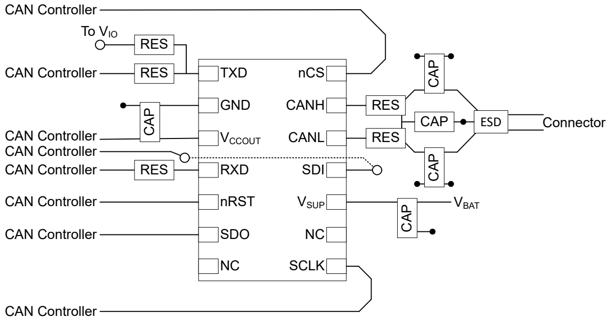
图 9-4. TCAN1164 示例布局
