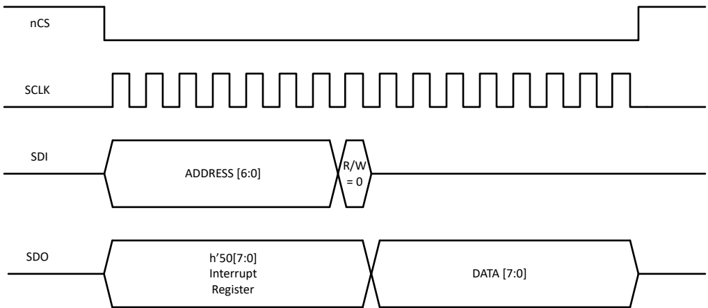
图 8-20. SPI 读取
