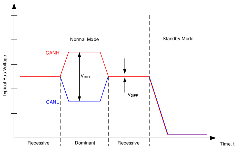
图 8-16. 总线状态
