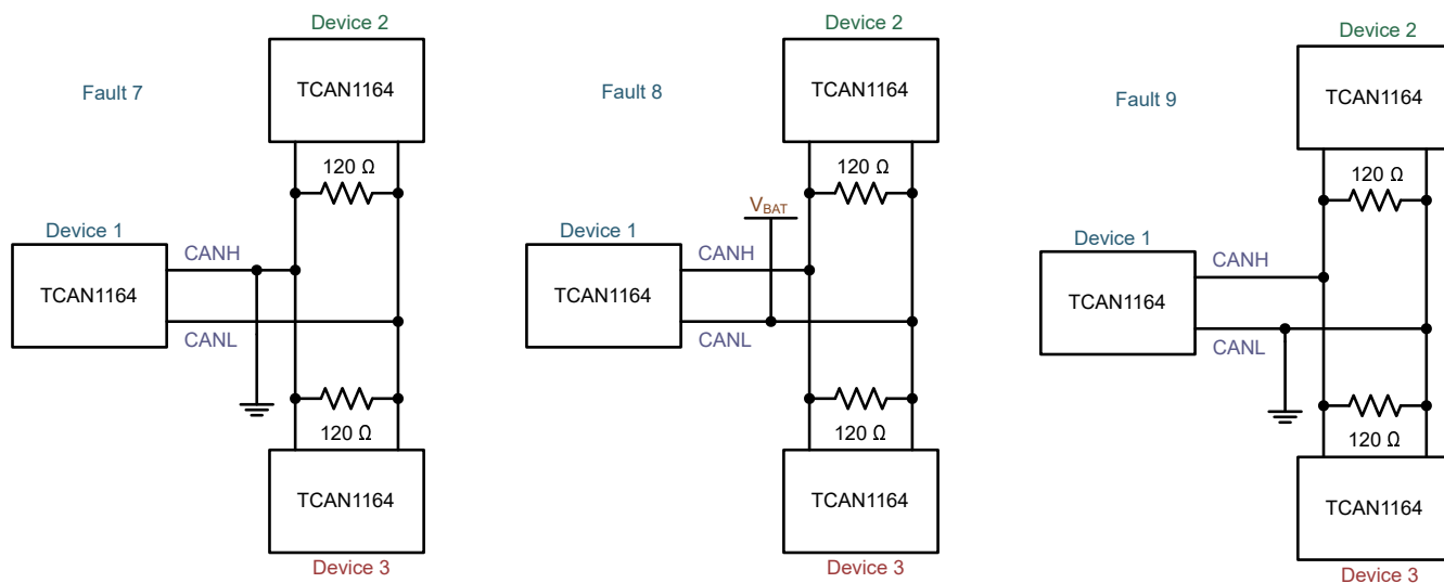
图 8-11. 故障 7、8 和 9 示例
