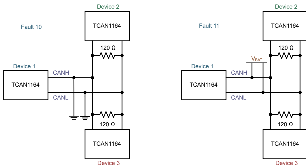
图 8-12. 故障 10 和 11 示例
