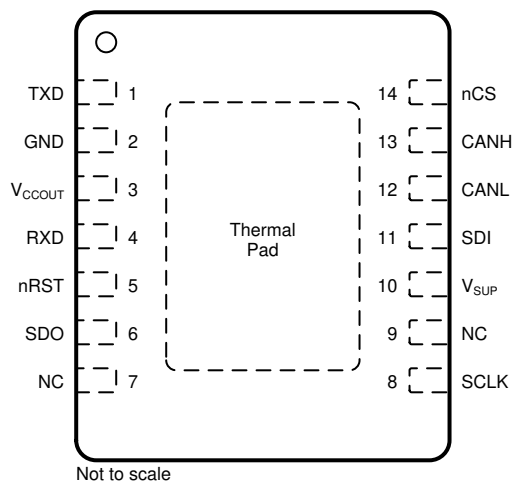
图 5-1. DMT 封装，14 引脚 (VSON) (顶视图)
