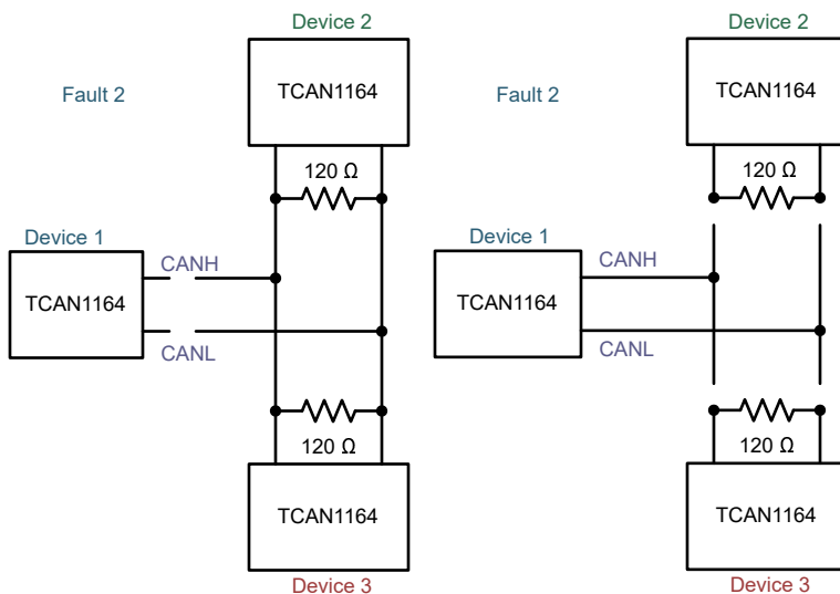
图 8-7. 三节点示例
