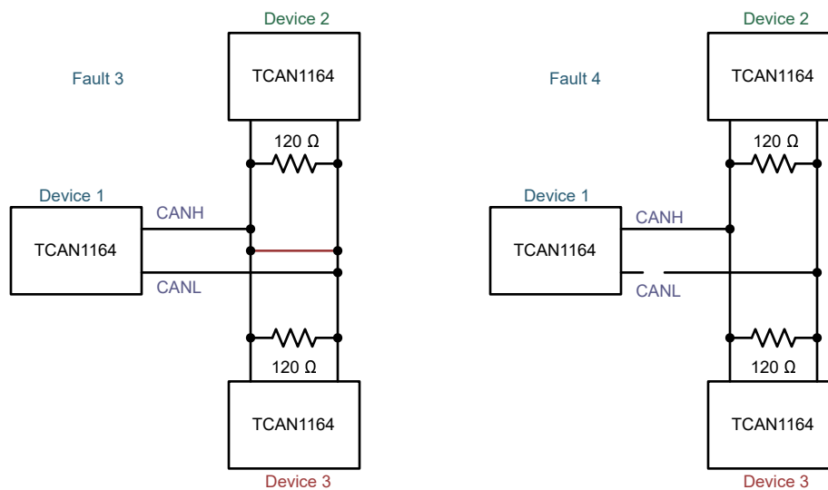
图 8-9. 故障 3 和 4 示例
