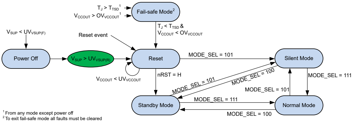
图 8-13. TCAN1164 状态机
