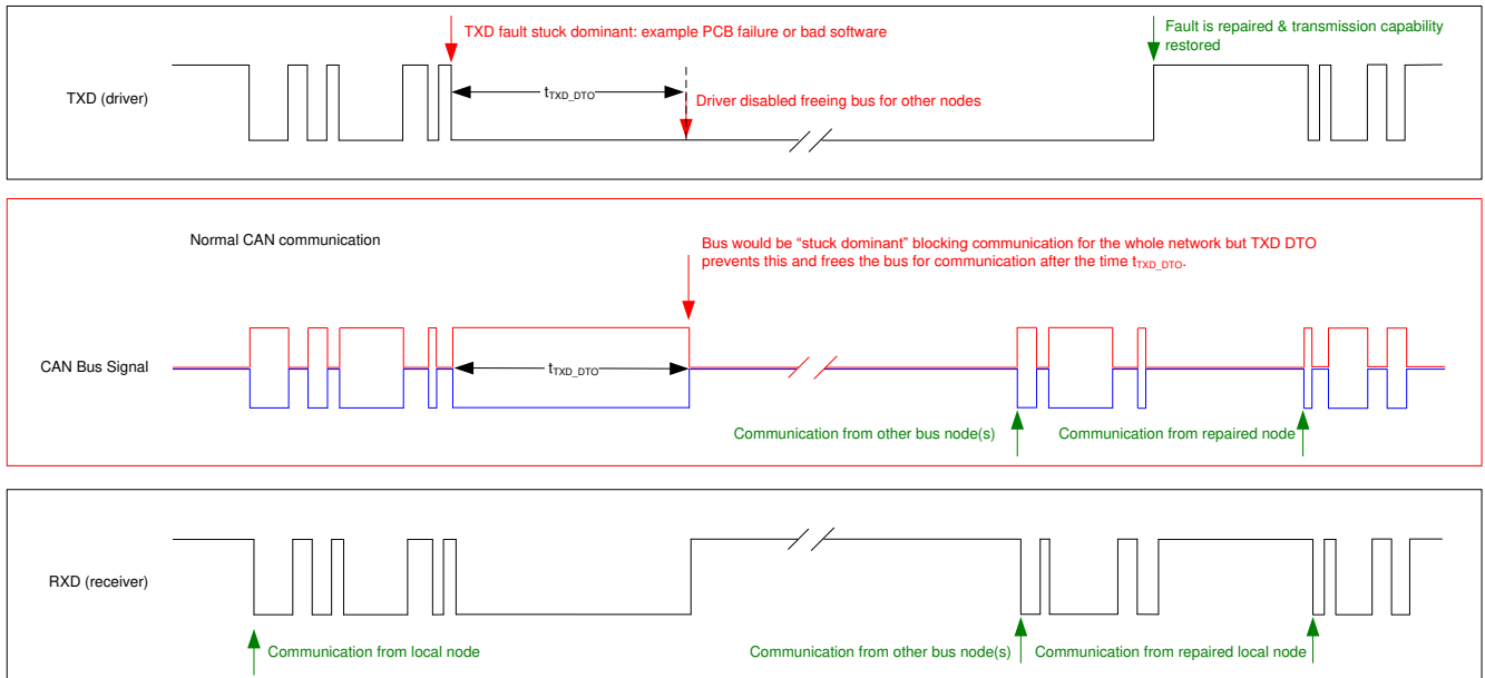
图 8-2. TXD DTO 的时序图
