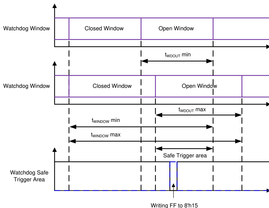
图 8-3. 窗口看门狗时序图
