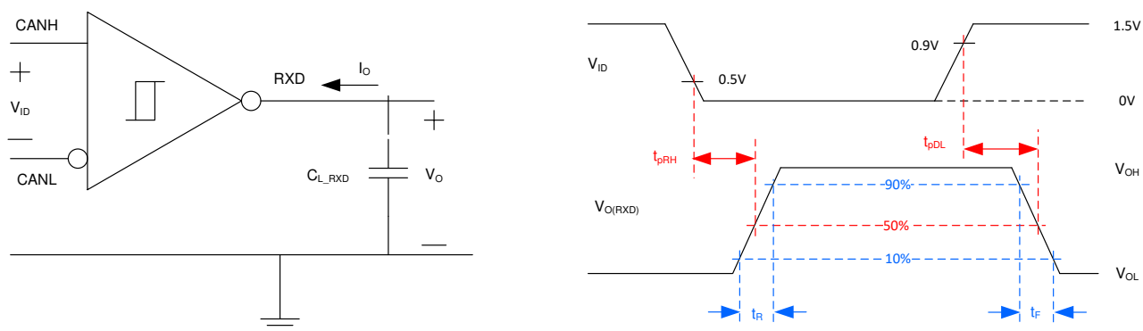
图 7-3. 接收器测试电路与测量
