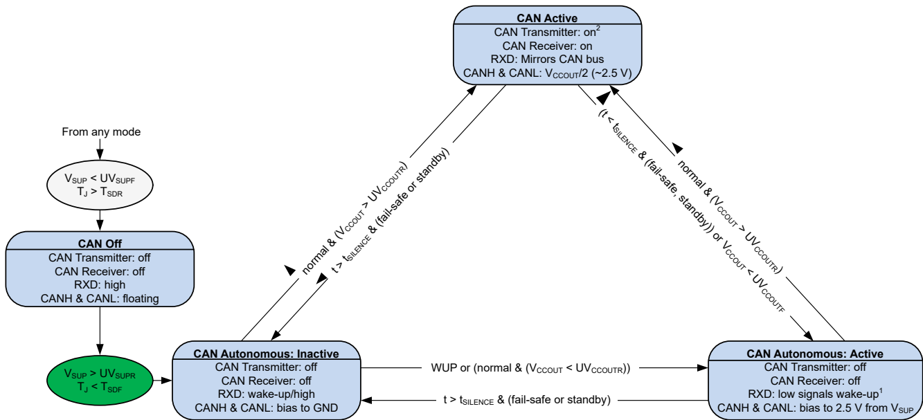
图 8-15. TCAN1164 CAN 收发器状态机
