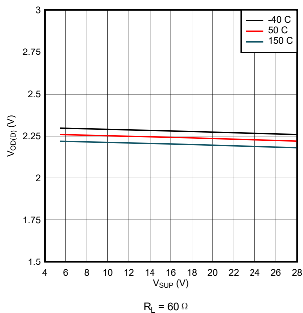
图 9-3. V_{OD(D)} 与 V_{SUP} 之间的关系
