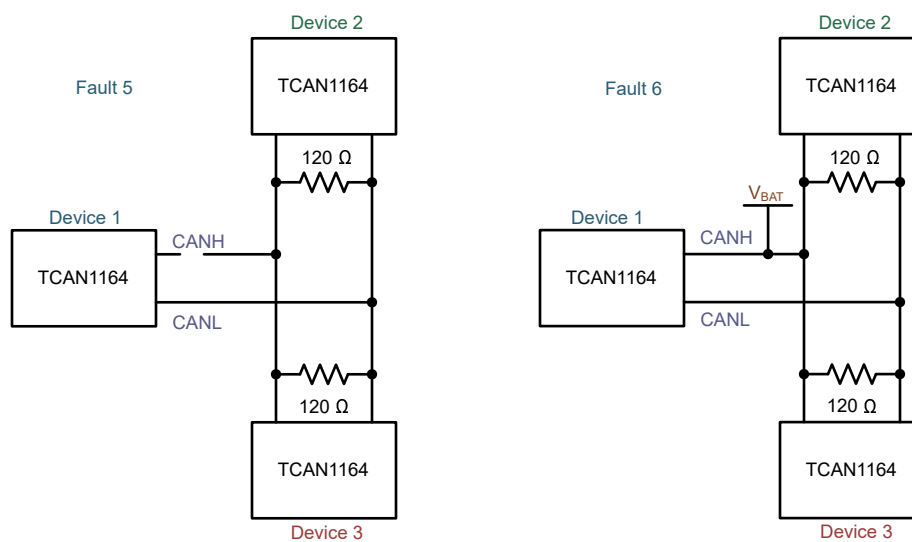
图 8-10. 故障 5 和 6 示例
