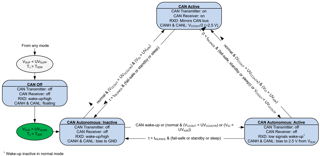
图 7-12. TCAN11625 CAN 收发器状态机
