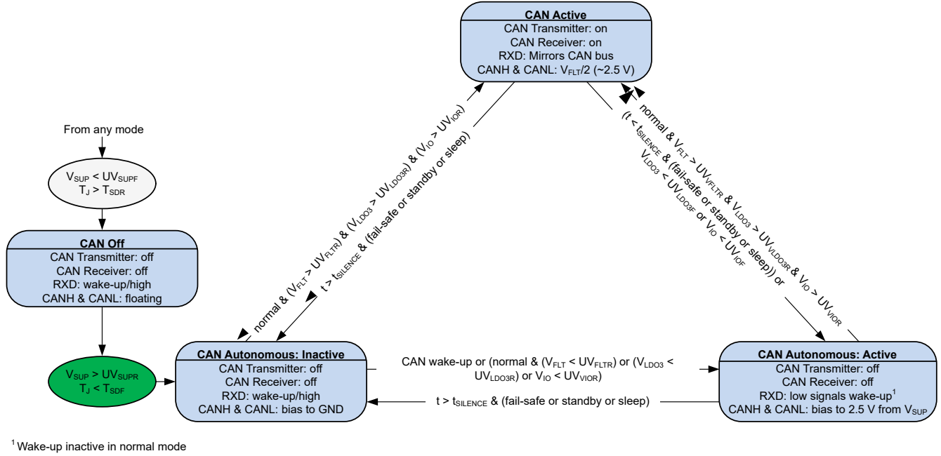
图 7-11. TCAN11623 CAN 收发器状态机
