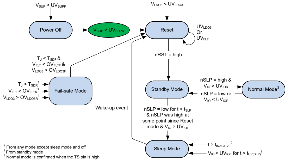
图 7-5. TCAN11623 状态机
