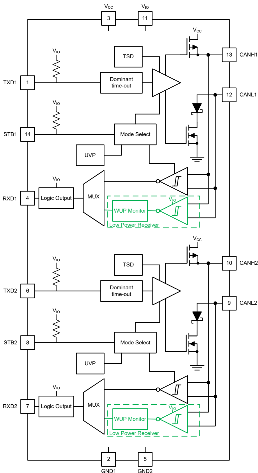
图 8-1. Block Diagram
