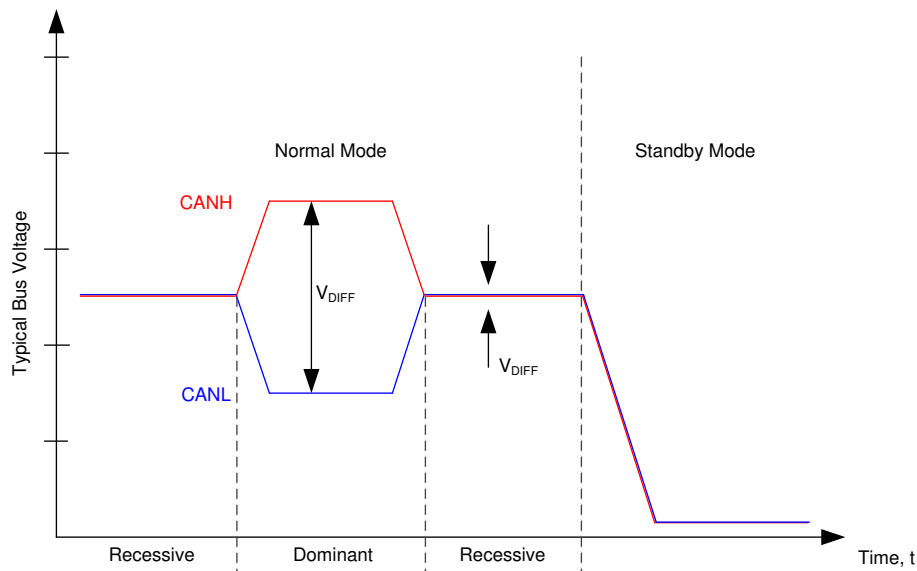
图 8-2. Bus States
