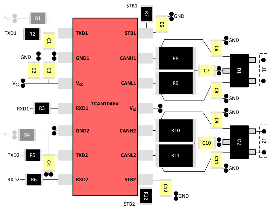
图 11-1. Example Layout
