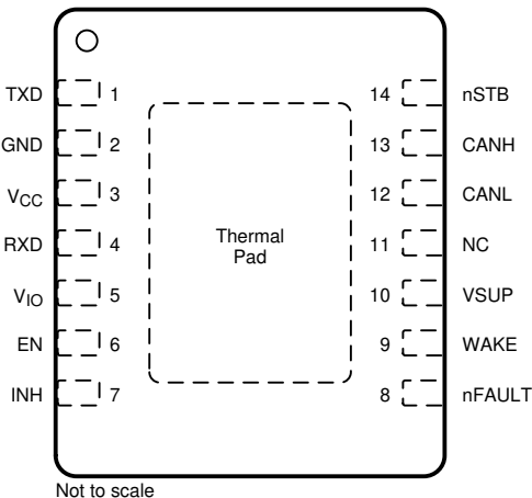
图 5-2. DMT Package, 14 Pin (VSON) (Top View)
