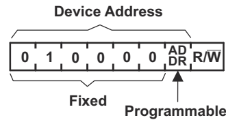
图 7-7. TCAL6416R 地址
