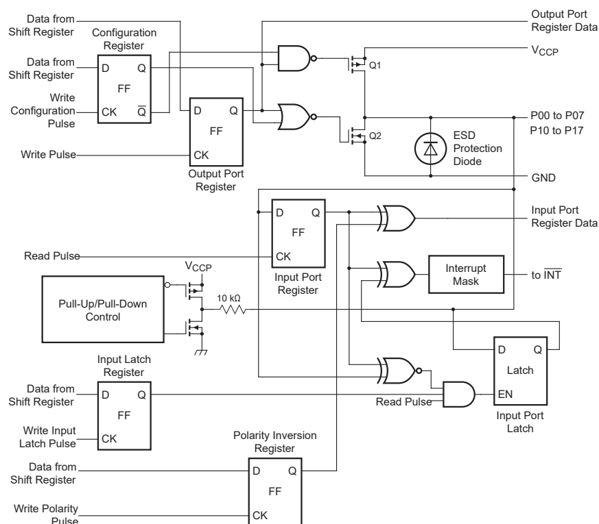
图 7-1. 逻辑图 (正逻辑)
