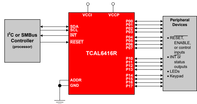
简化原理图
