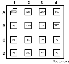
图 4-3. DTU (X2QFN) 封装，16 引脚 (俯视图)
