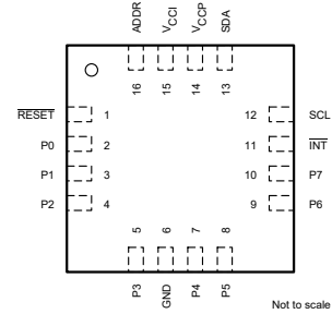
图 4-2. RSV (UQFN) 封装，16 引脚 (俯视图)
