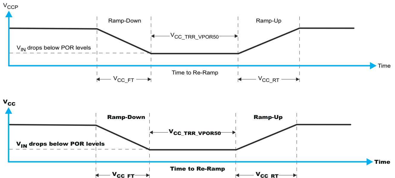
图 8-7. 将 V_{CCP} 降至低于 POR 阈值，然后重新斜升
