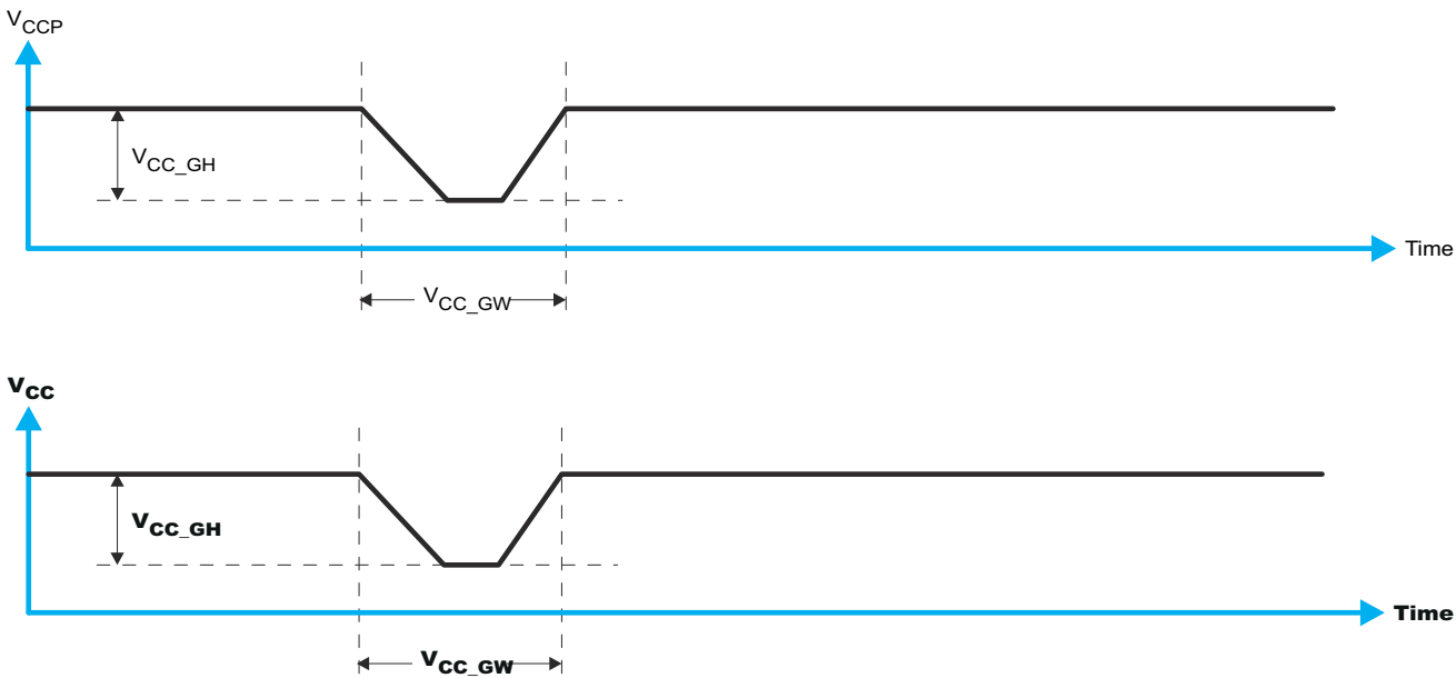
图 8-8. 干扰宽度和干扰高度
