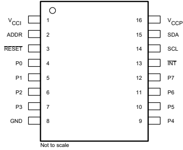
图 4-1. PW (TSSOP) 封装，16 引脚 (俯视图)
