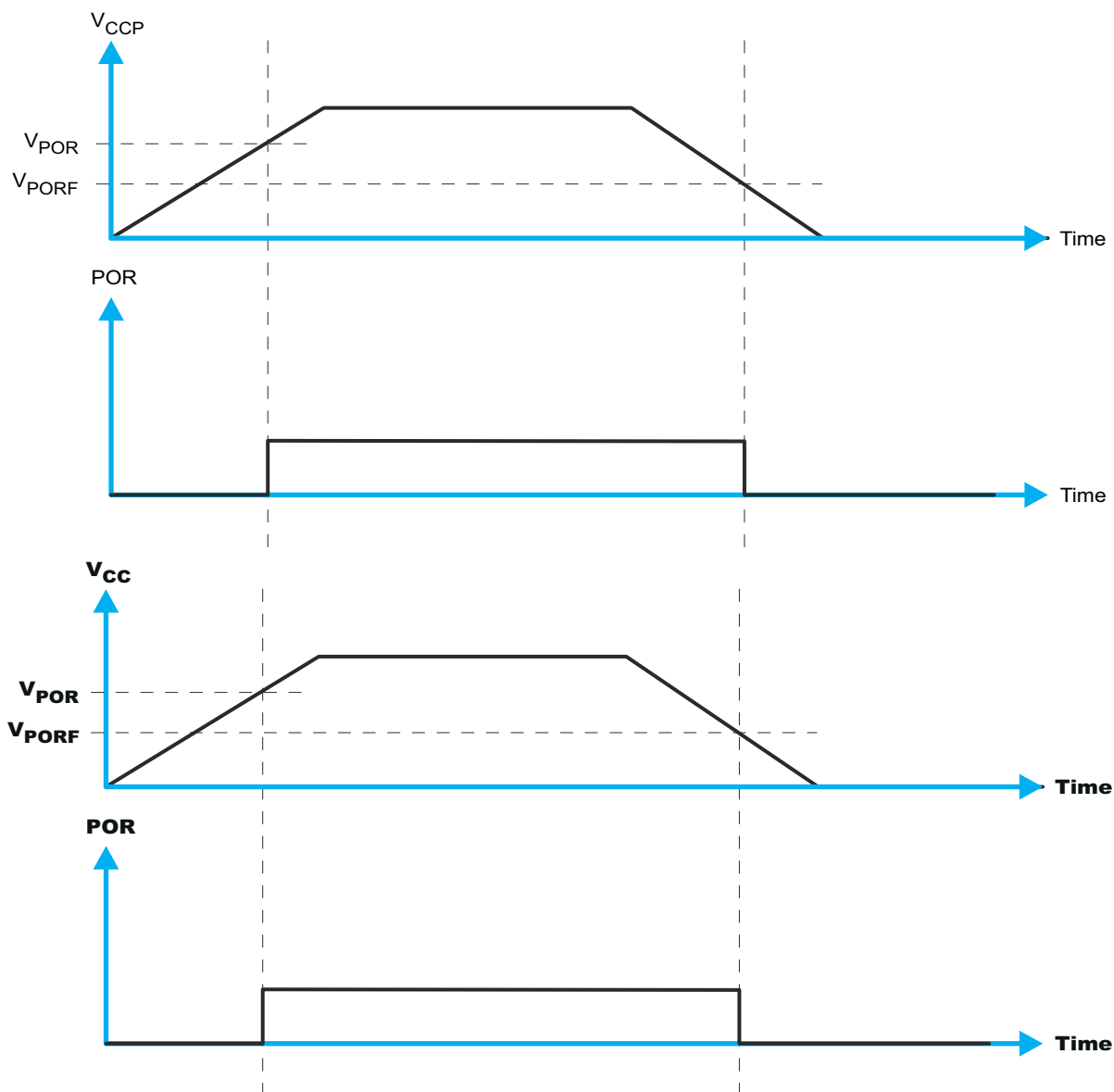
图 8-9. V_{POR}
