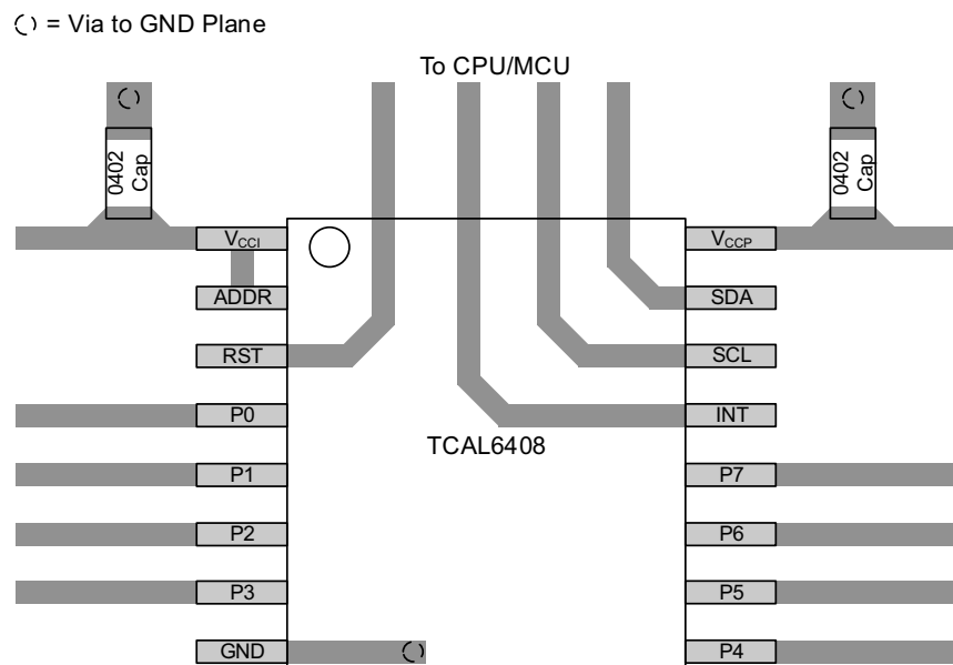
图 8-10. TCAL6408 布局
