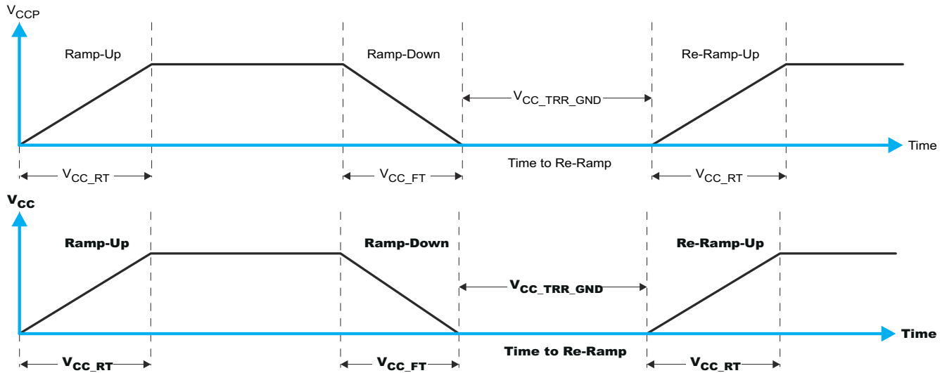
图 8-6. 将 V_{CCP} 降至 0.2V 或 0V 以下，然后斜升
