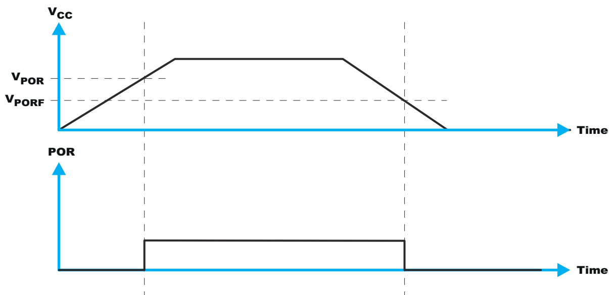
图 10-4. V_{POR}
