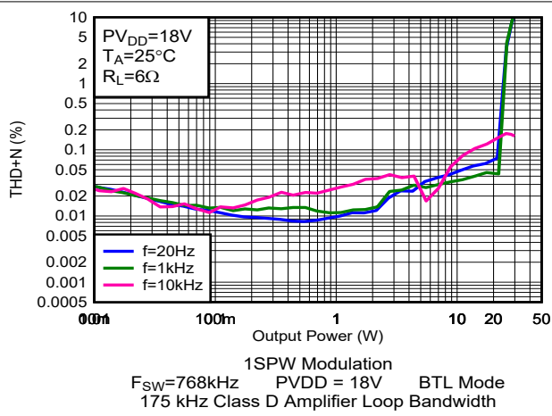
图 5-63. THD+N 与输出功率间的关系
