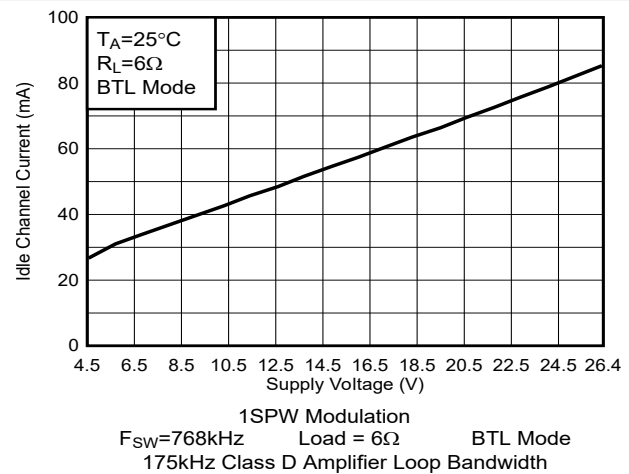
图 5-81. PVDD 空闲电流与 PVDD 电压间的关系
