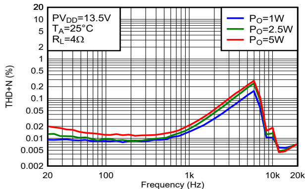
图 5-1. THD+N 与频率间的关系
