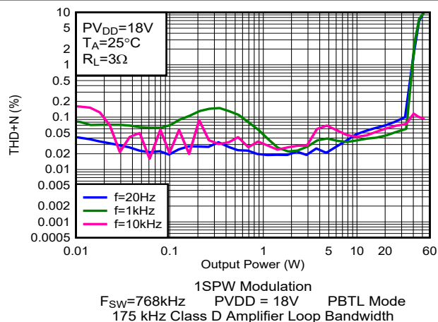
图 5-103. THD+N 与输出功率间的关系
