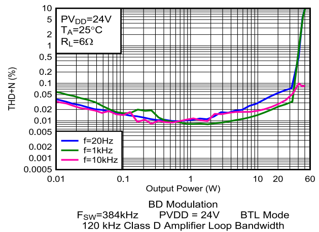
图 5-22. THD+N 与输出功率间的关系
