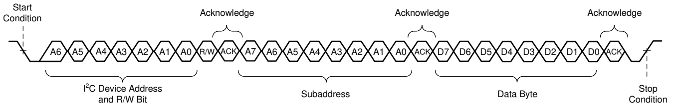
图 6-10. 随机写入传输
