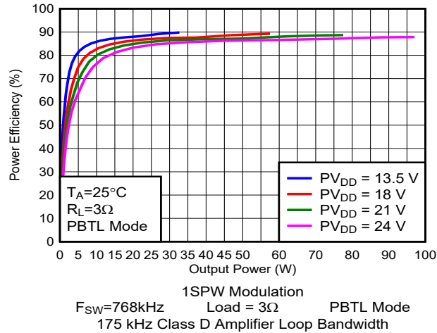
图 5-110. 效率与输出功率间的关系
