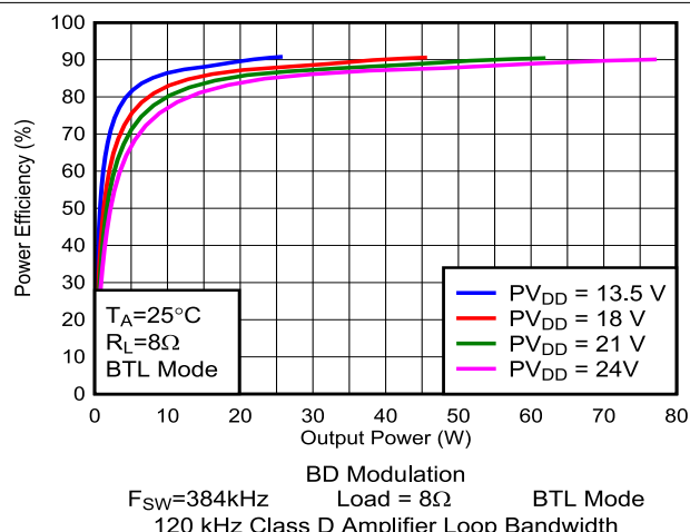
图 5-42. 效率与输出功率间的关系
