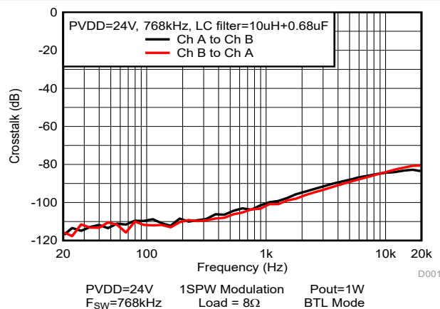
图 5-80. 串扰
