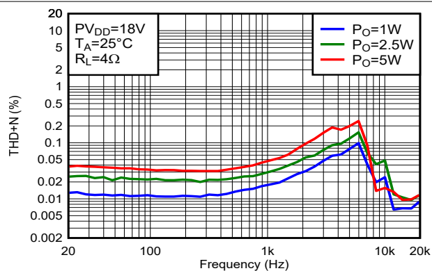
图 5-47. THD+N 与频率间的关系
