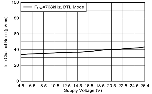
图 5-73. 空闲声道噪声与电源电压间的关系
