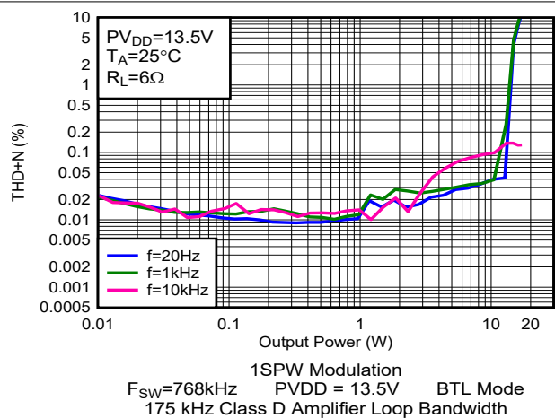
图 5-62. THD+N 与输出功率间的关系
