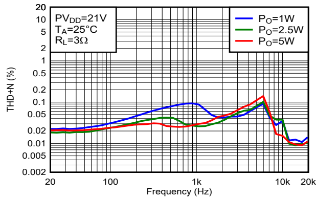
图 5-98. THD+N 与频率间的关系
