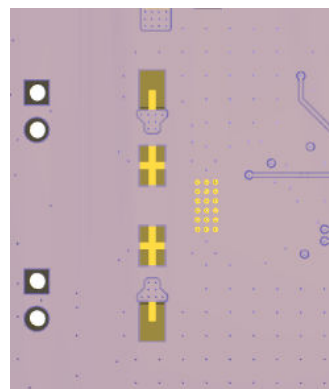
Bot Layer Layout
