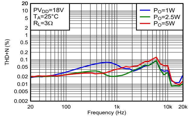
图 5-99. THD+N 与频率间的关系
