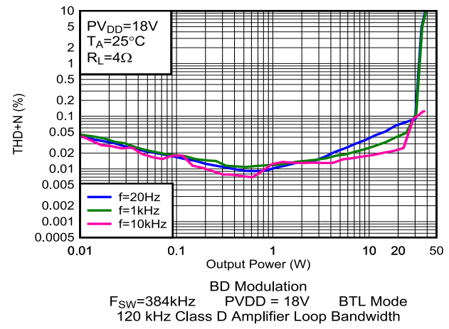
图 5-16. THD+N 与输出功率间的关系
