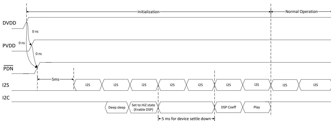
图 6-14. 启动顺序
