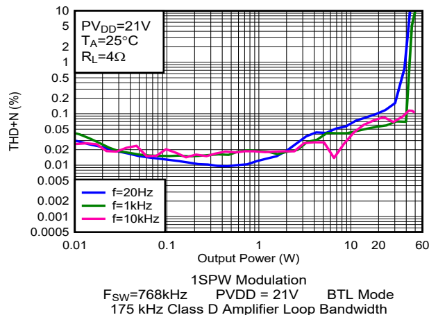
图 5-60. THD+N 与输出功率间的关系
