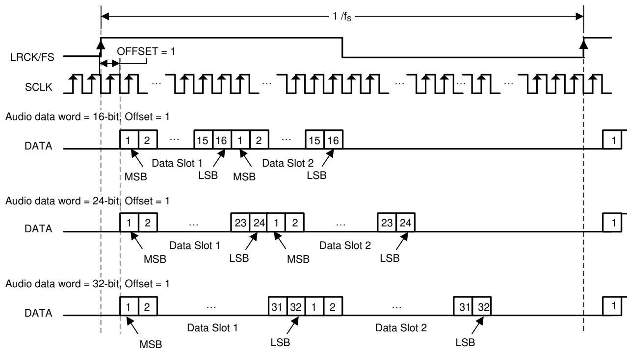
图 6-5. TDM 1 音频数据格式
