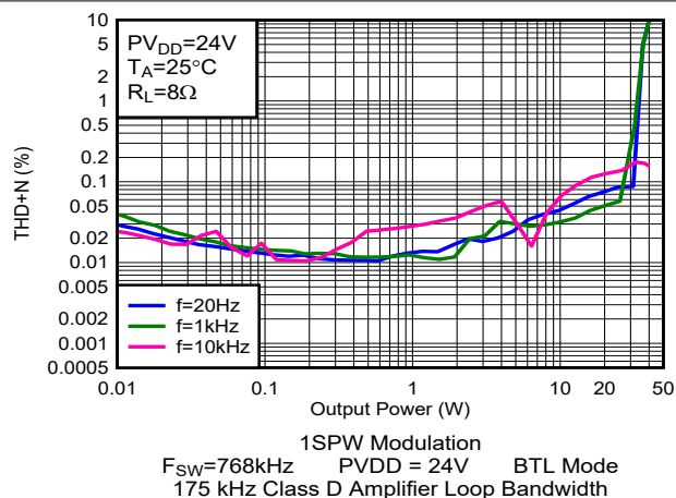
图 5-69. THD+N 与输出功率间的关系
