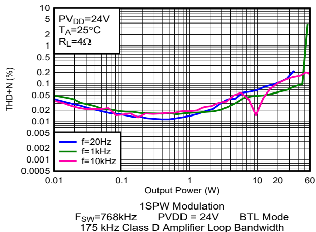
图 5-61. THD+N 与输出功率间的关系
