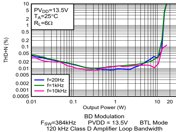
图 5-19. THD+N 与输出功率间的关系
