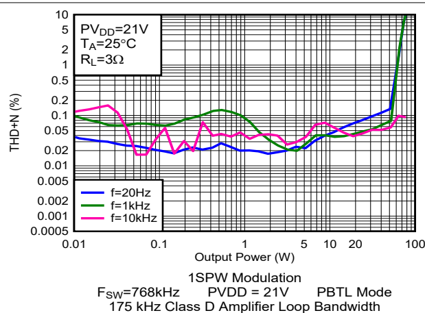
图 5-104. THD+N 与输出功率间的关系
