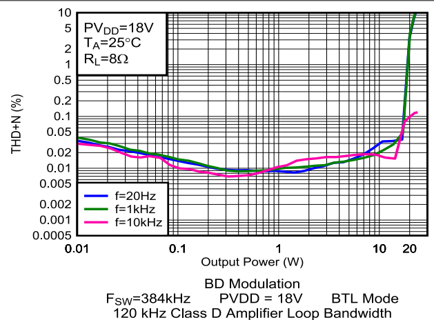
图 5-24. THD+N 与输出功率间的关系
