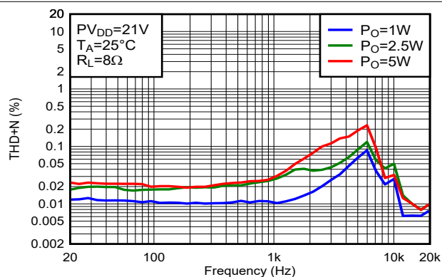
图 5-54. THD+N 与频率间的关系
