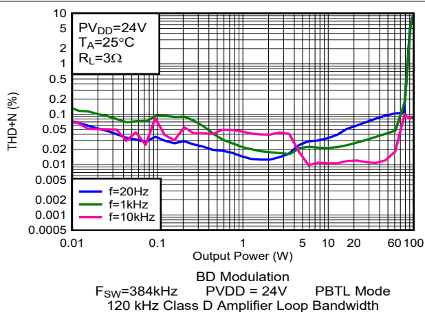
图 5-92. THD+N 与输出功率间的关系
