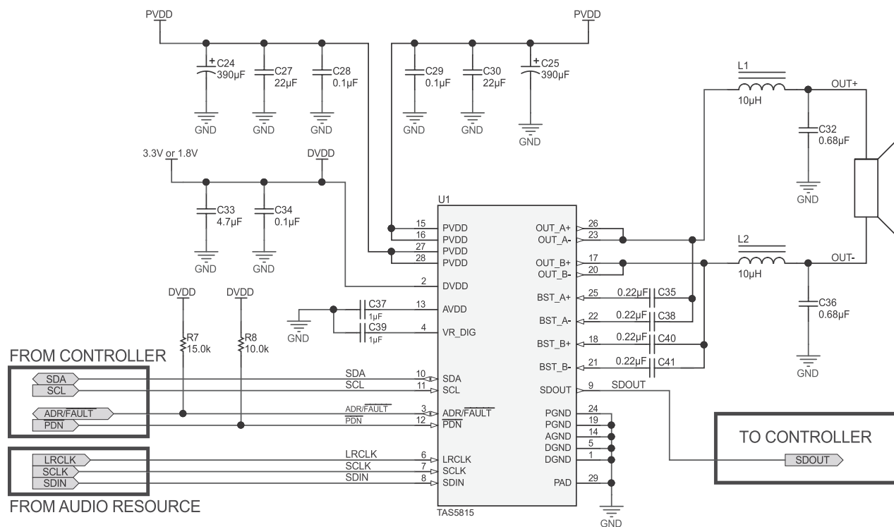
图 8-3. 单声道 (PBTL) 系统应用原理图
