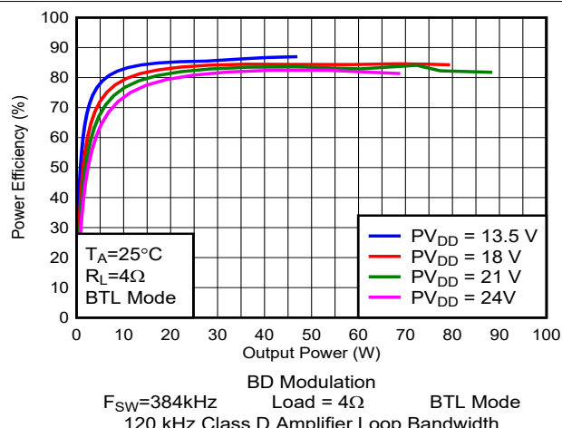
图 5-40. 效率与输出功率间的关系
