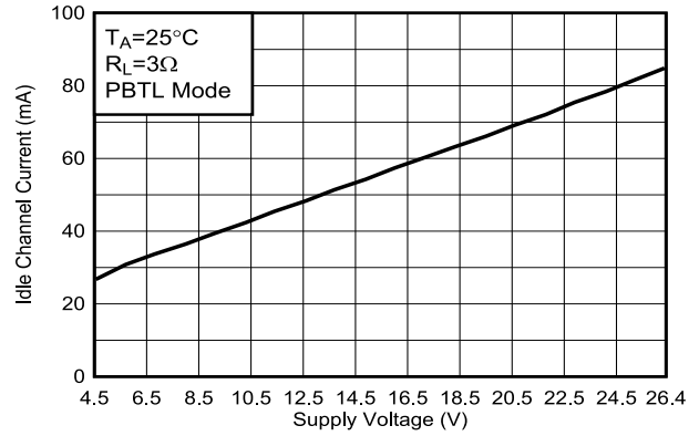
图 5-109. PV_{DD} 空闲电流与 PV_{DD} 电压间的关系
