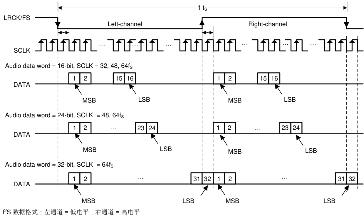
图 6-3. I²S 音频数据格式
