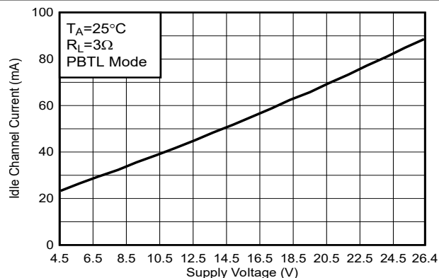
图 5-96. PVDD 空闲电流与 PVDD 电压间的关系
