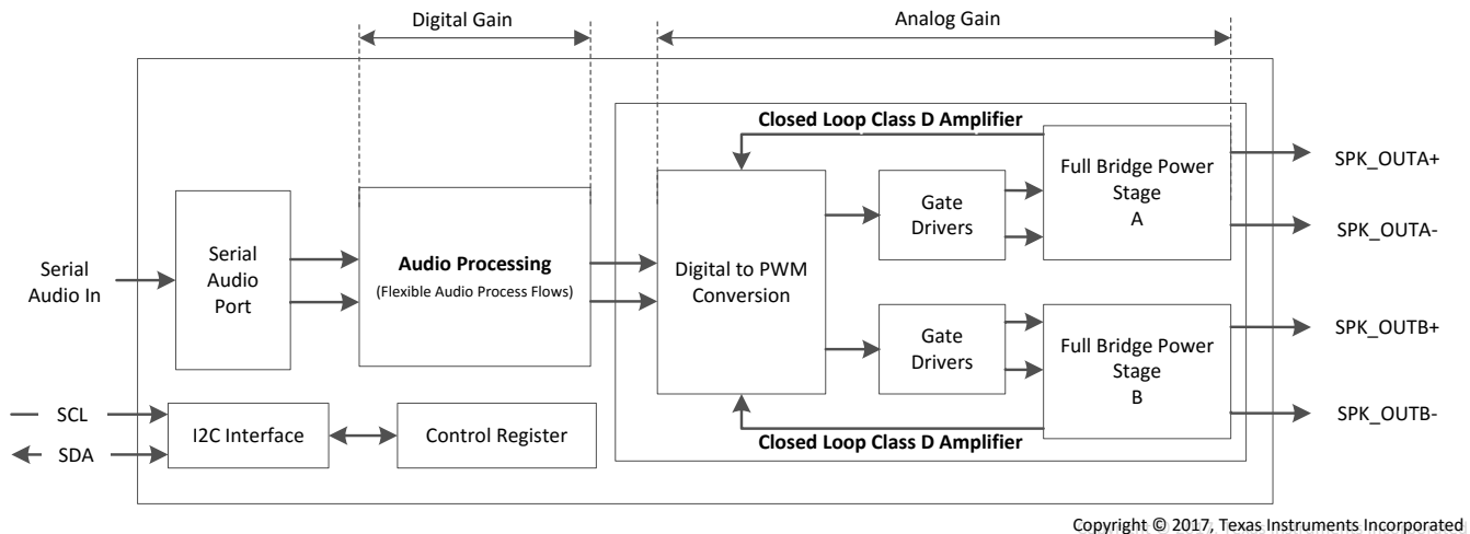
图 6-7. 扬声器放大器增益
