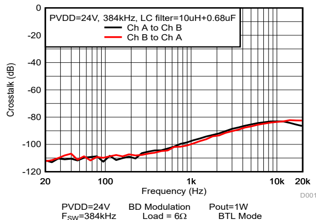
图 5-37. 串扰
