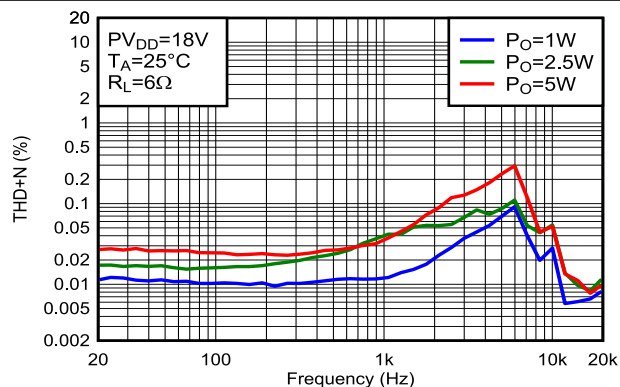
图 5-49. THD+N 与频率间的关系
