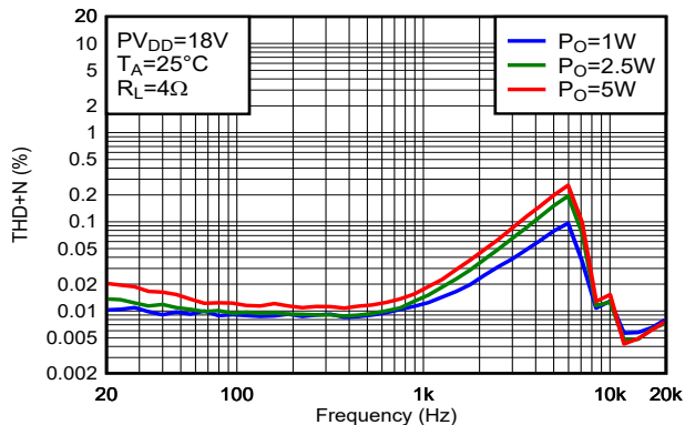
图 5-2. THD+N 与频率间的关系
