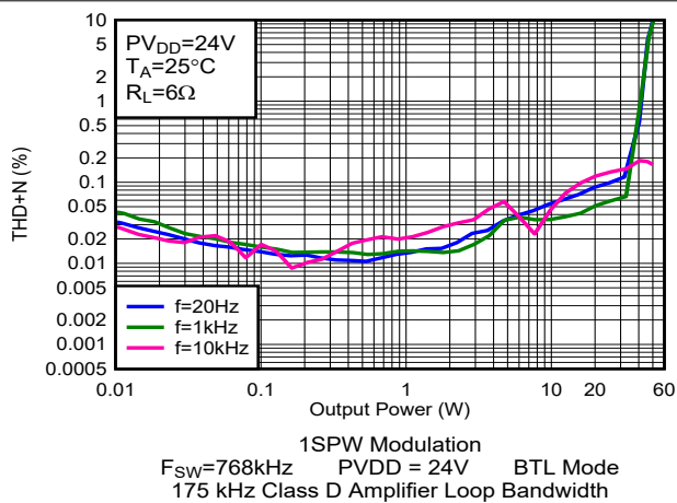
图 5-65. THD+N 与输出功率间的关系
