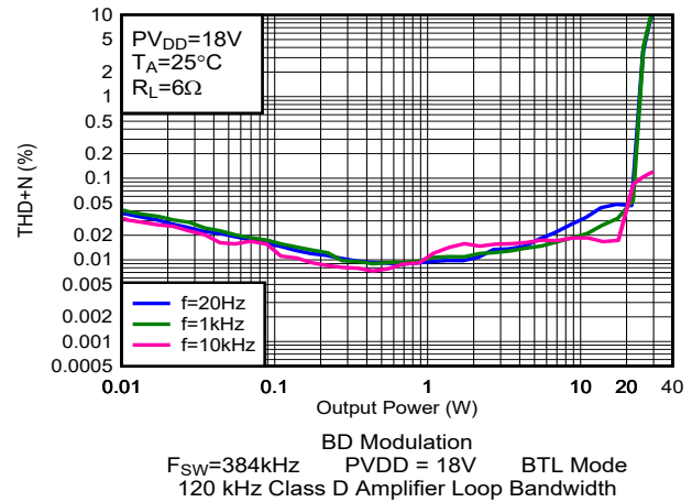
图 5-20. THD+N 与输出功率间的关系
