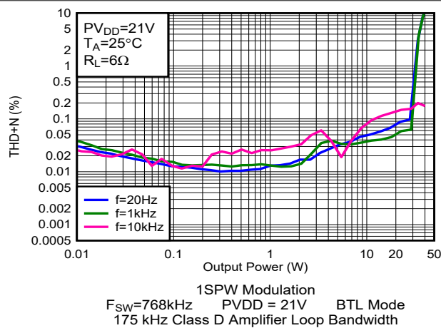
图 5-64. THD+N 与输出功率间的关系
