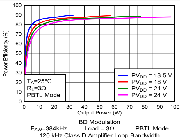
图 5-97. 效率与输出功率间的关系
