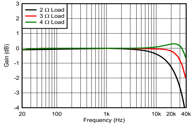
图 5-108. 增益与频率间的关系
