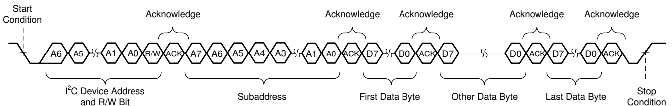
图 6-12. 顺序写入传输
