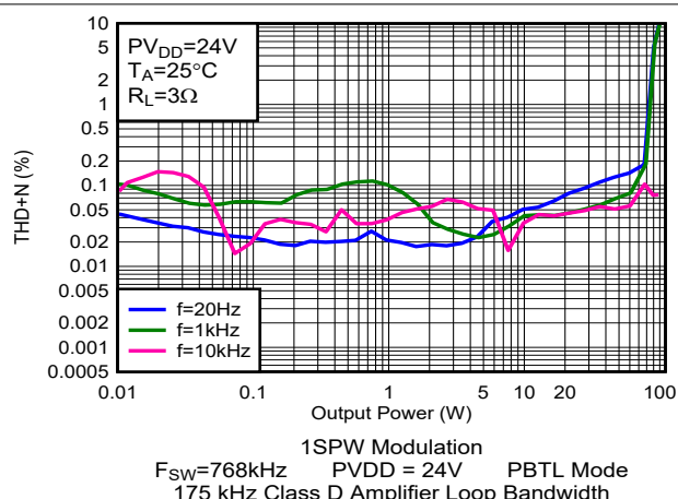
图 5-105. THD+N 与输出功率间的关系
