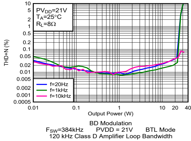
图 5-25. THD+N 与输出功率间的关系
