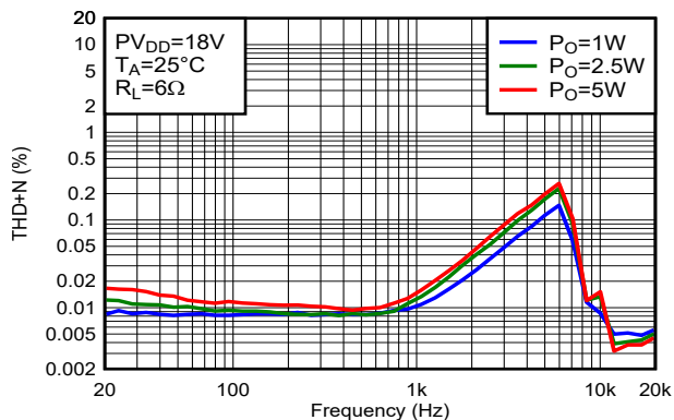
图 5-4. THD+N 与频率间的关系
