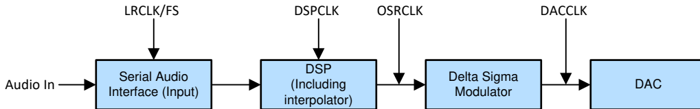
图 6-1. 具有相应时钟的音频流
