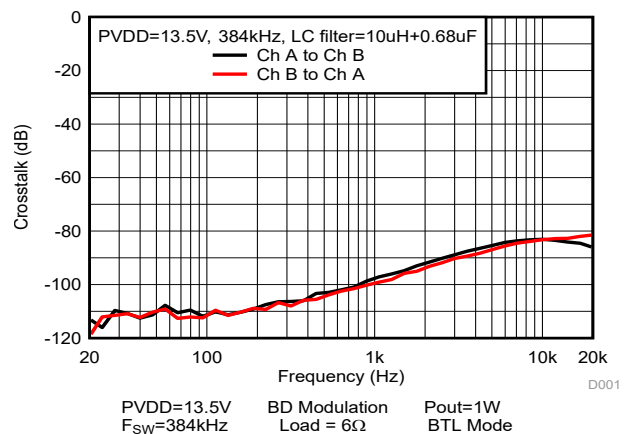
图 5-36. 串扰
