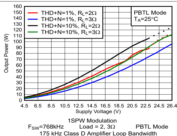
图 5-106. 输出功率与电源电压间的关系 (虚线表示热限制)
