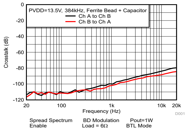
图 5-38. 串扰
