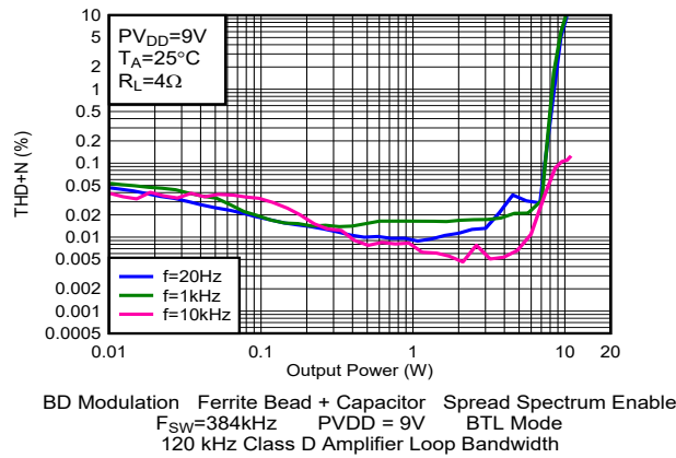
图 5-27. THD+N 与输出功率间的关系
