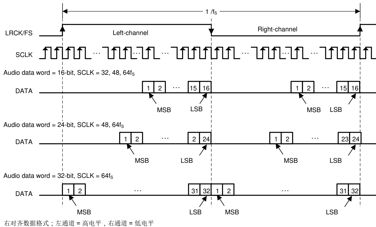
图 6-4. 右对齐音频数据格式
