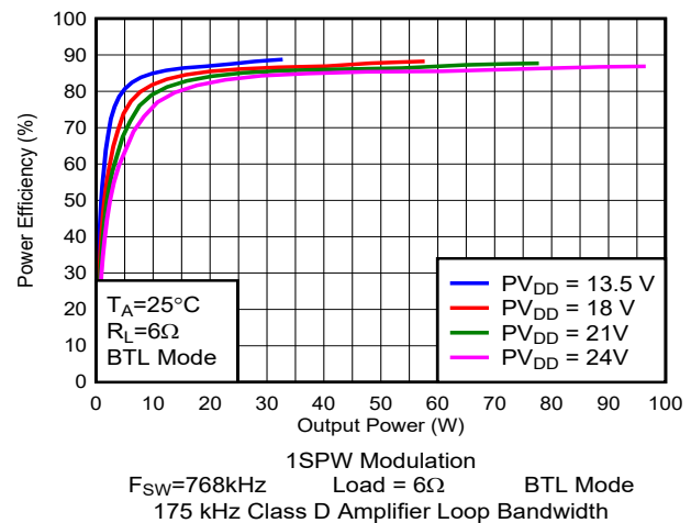
图 5-83. 效率与输出功率间的关系
