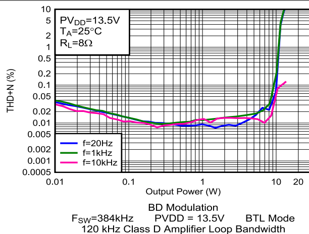
图 5-23. THD+N 与输出功率间的关系
