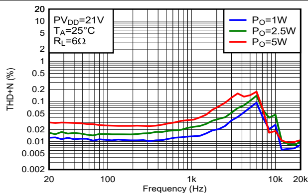
图 5-50. THD+N 与频率间的关系
