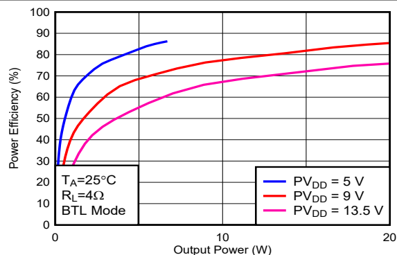
图 5-43. 效率与输出功率间的关系 (带 FB)
