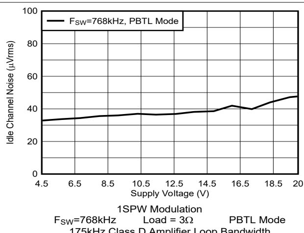
图 5-107. 空闲声道噪声与电源电压间的关系
