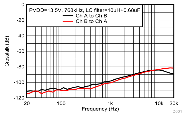
图 5-77. 串扰
