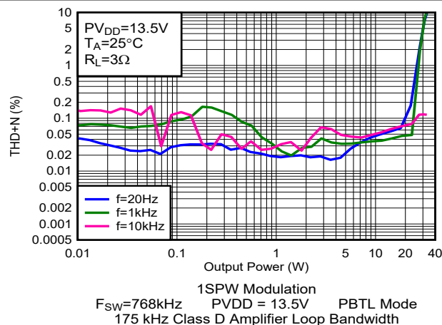
图 5-102. THD+N 与输出功率间的关系
