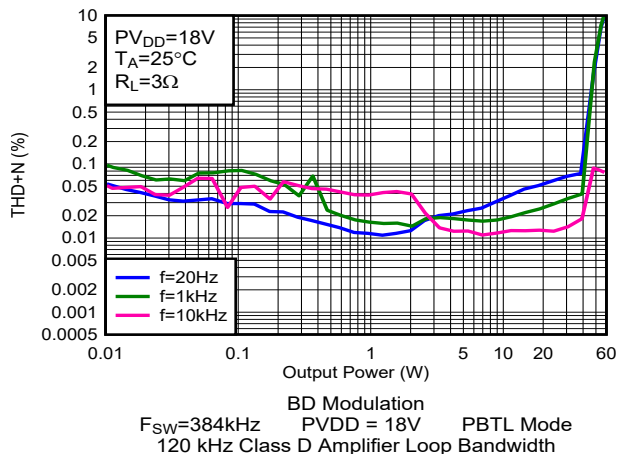
图 5-90. THD+N 与输出功率间的关系
