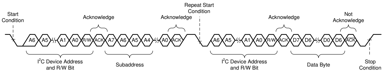
图 6-11. 随机读取传输
