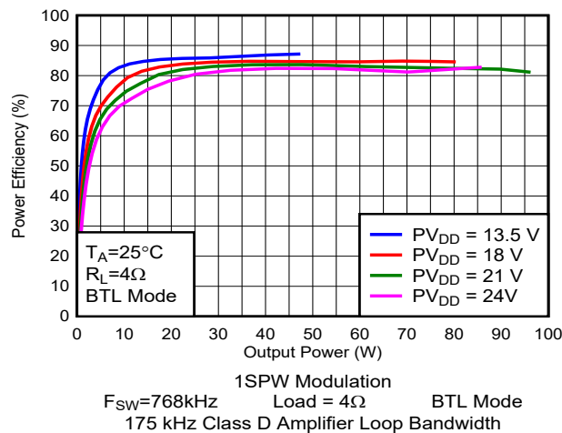
图 5-82. 效率与输出功率间的关系
