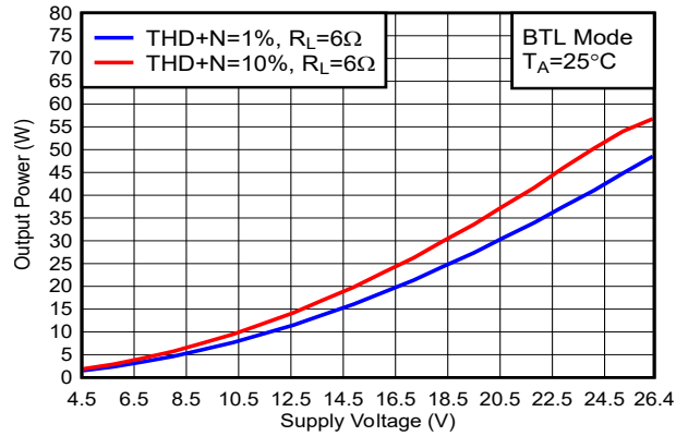
图 5-31. 输出功率与电源电压间的关系
