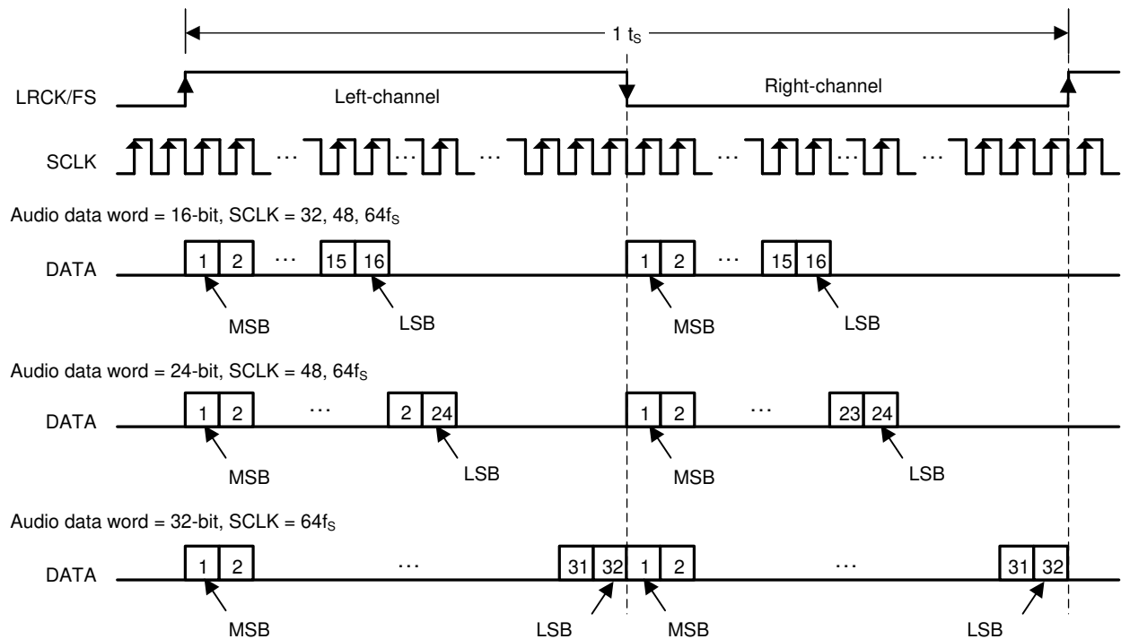
图 6-2. 左对齐音频数据格式
