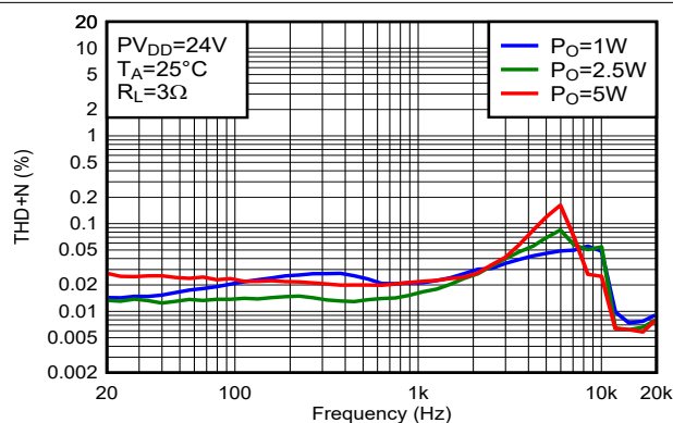
图 5-86. THD+N 与频率间的关系
