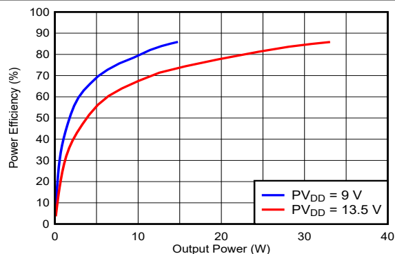
图 5-44. 效率与输出功率间的关系
