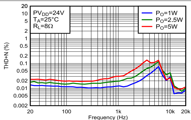
图 5-55. THD+N 与频率间的关系
