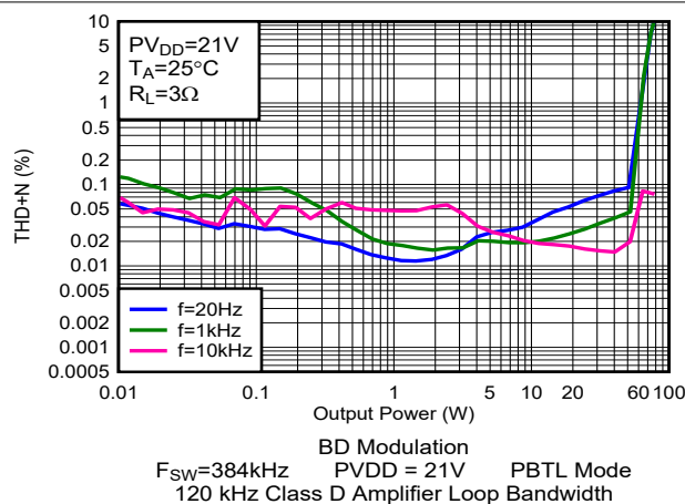
图 5-91. THD+N 与输出功率间的关系
