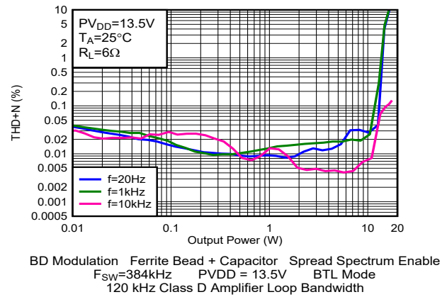
图 5-28. THD+N 与输出功率间的关系
