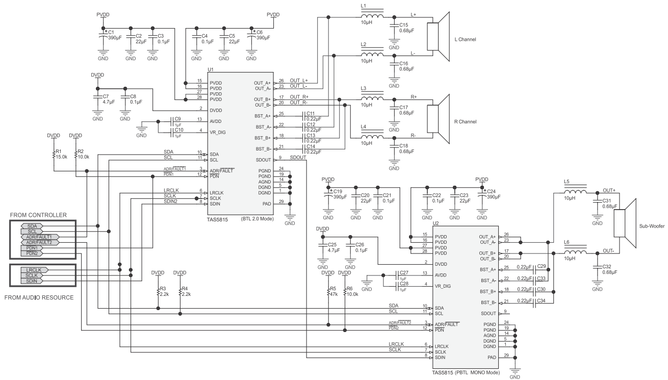
图 8-4. 2.1（带两个 TAS5815 器件的 2.1 通道）应用原理图
