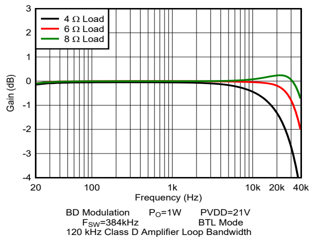
图 5-35. 增益与频率间的关系
