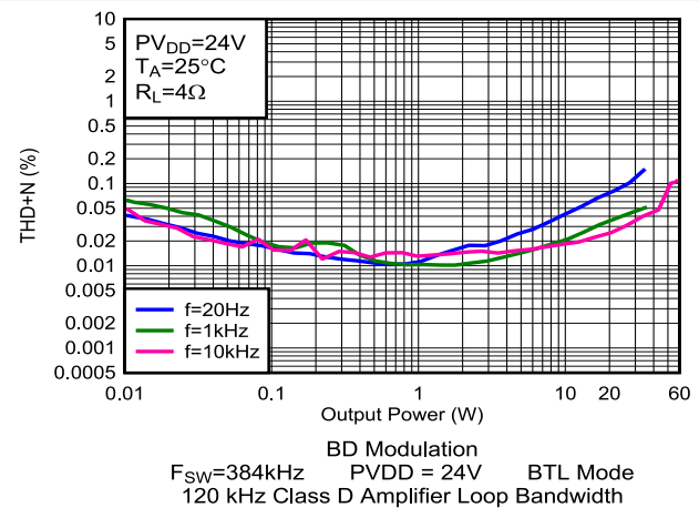
图 5-18. THD+N 与输出功率间的关系
