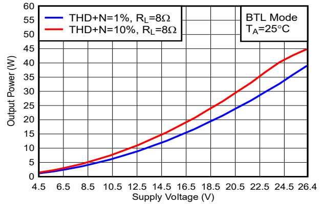
图 5-32. 输出功率与电源电压间的关系
