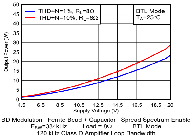
图 5-33. 输出功率与电源电压间的关系
