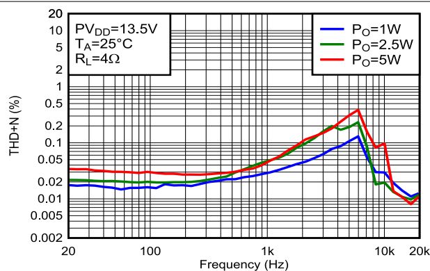
图 5-46. THD+N 与频率间的关系
