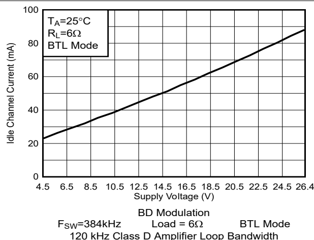
图 5-39. PVDD 空闲电流与 PVDD 电压间的关系
