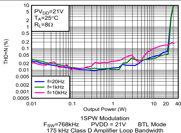
图 5-68. THD+N 与输出功率间的关系
