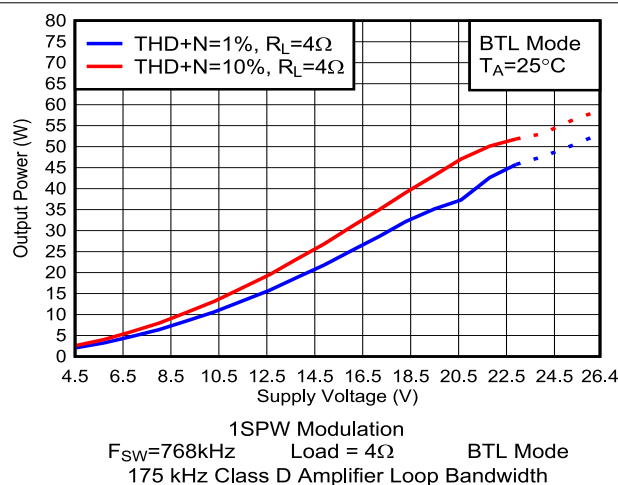
图 5-70. 输出功率与电源电压间的关系 (虚线表示热限制)
