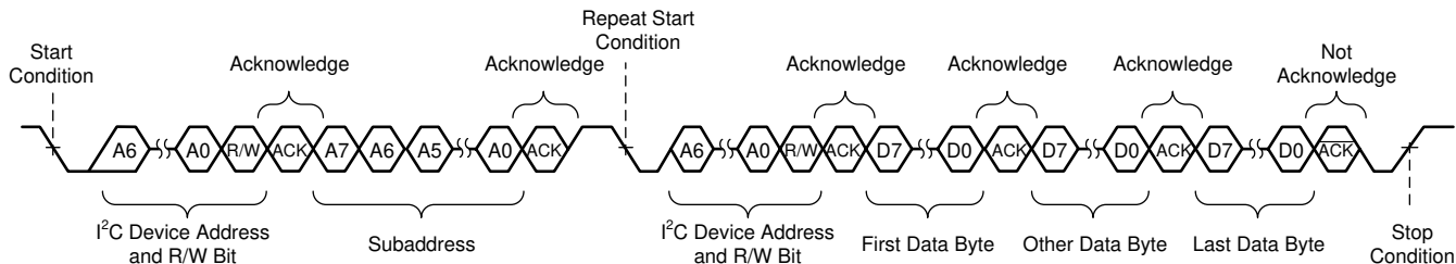
图 6-13. 顺序读取传输
