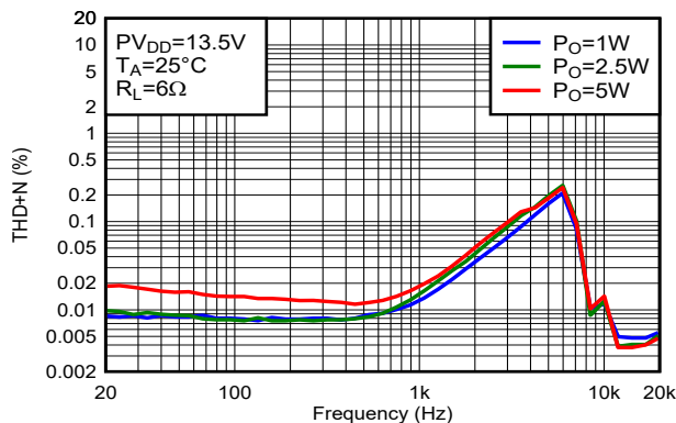
图 5-3. THD+N 与频率间的关系
