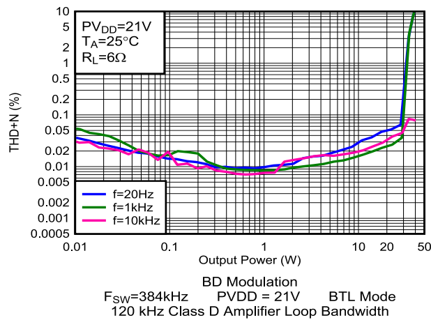
图 5-21. THD+N 与输出功率间的关系
