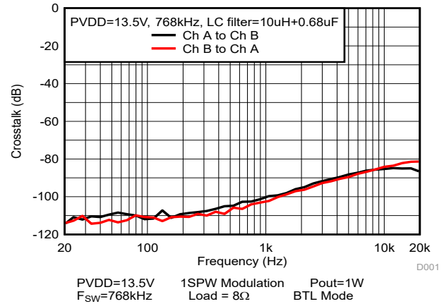
图 5-79. 串扰
