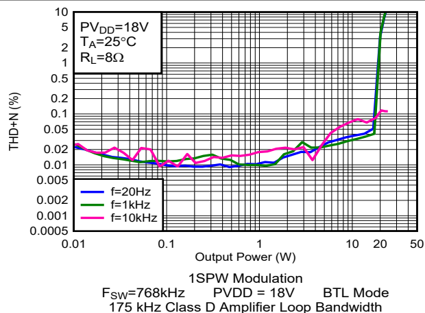
图 5-67. THD+N 与输出功率间的关系
