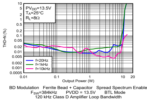
图 5-29. THD+N 与输出功率间的关系
