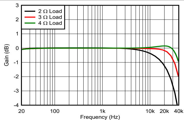
图 5-95. 增益与频率间的关系
