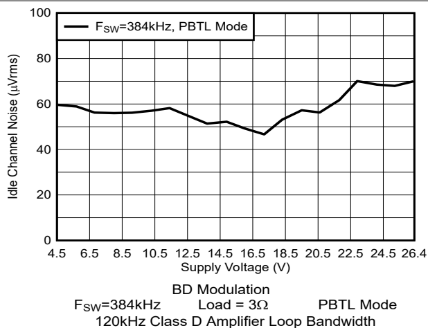
图 5-94. 空闲声道噪声与电源电压间的关系
