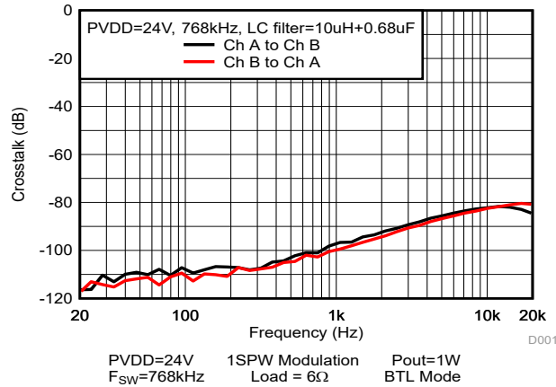
图 5-78. 串扰
