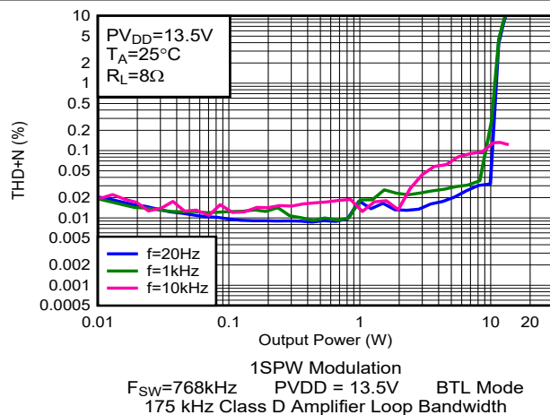
图 5-66. THD+N 与输出功率间的关系
