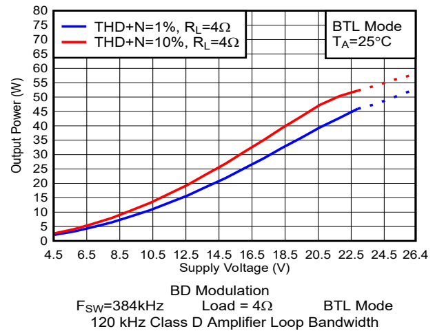
图 5-30. 输出功率与电源电压间的关系
