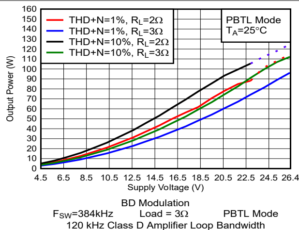
图 5-93. 输出功率与电源电压间的关系 (虚线表示热限制)
