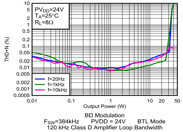
图 5-26. THD+N 与输出功率间的关系
