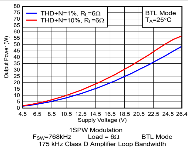
图 5-71. 输出功率与电源电压间的关系
