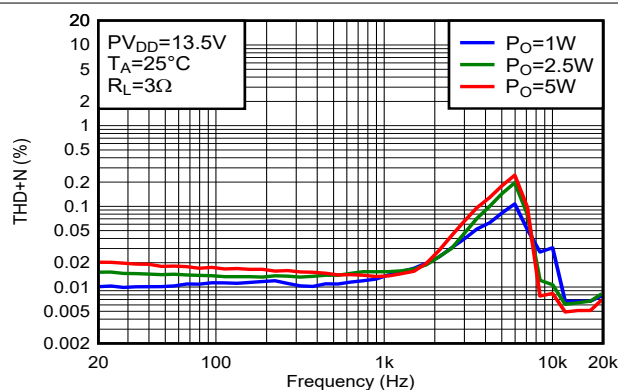
图 5-85. THD+N 与频率间的关系
