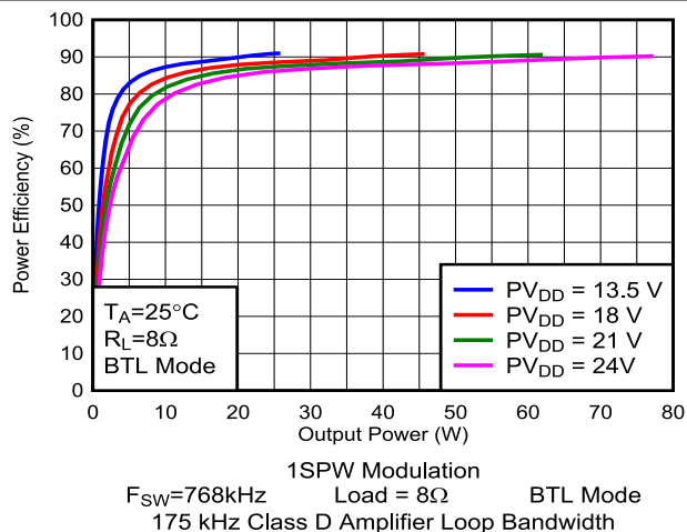
图 5-84. 效率与输出功率间的关系
