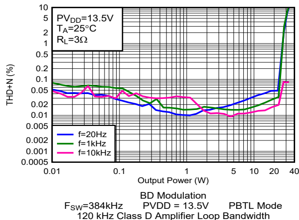
图 5-89. THD+N 与输出功率间的关系
