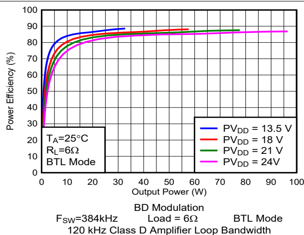
图 5-41. 效率与输出功率间的关系
