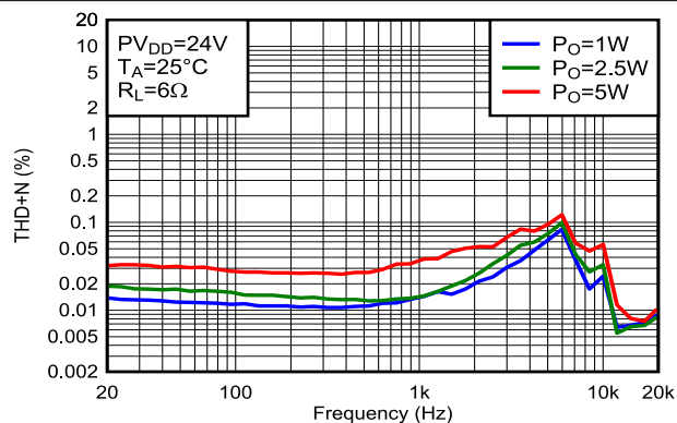
图 5-51. THD+N 与频率间的关系
