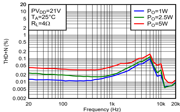
图 5-48. THD+N 与频率间的关系
