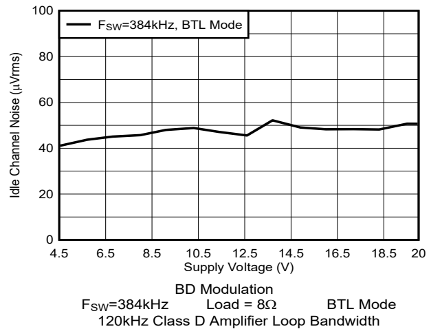
图 5-34. 空闲声道噪声与电源电压间的关系
