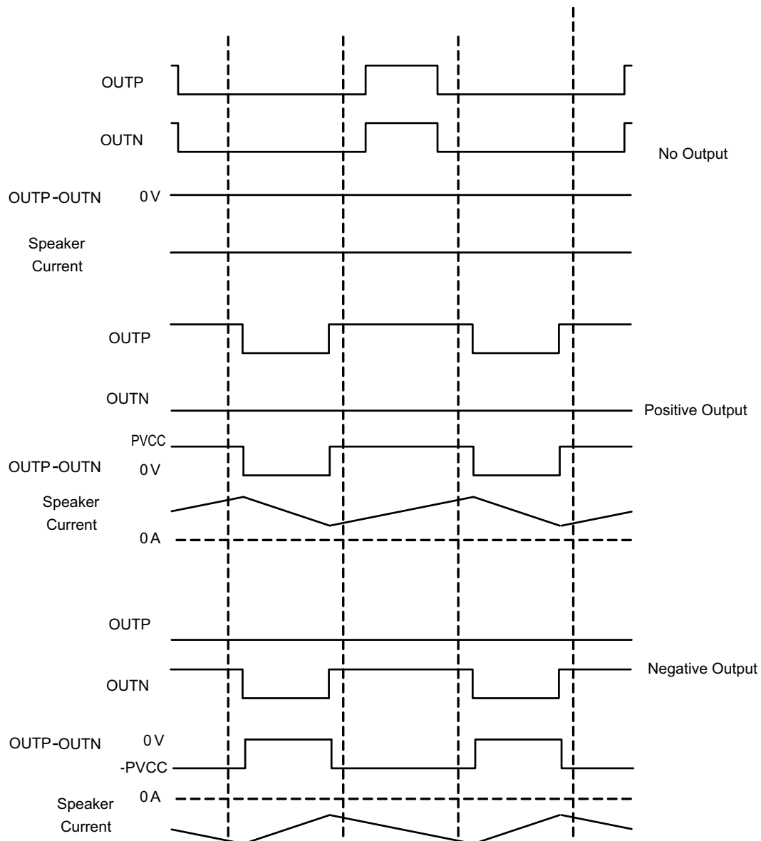
图 7-9. 1SPW Mode Modulation
