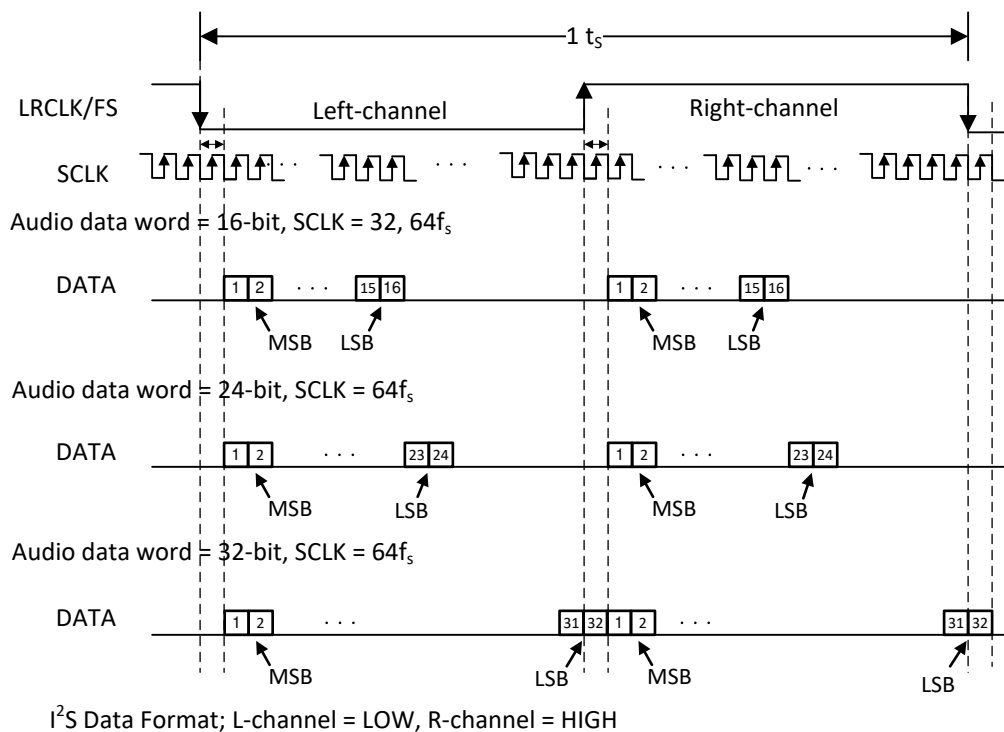
图 7-3. I²S Audio Data Format
