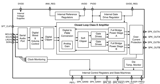
功能方框图
