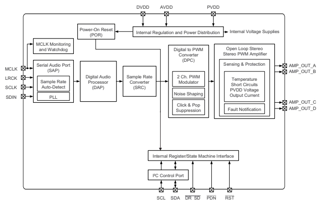
简化框图
