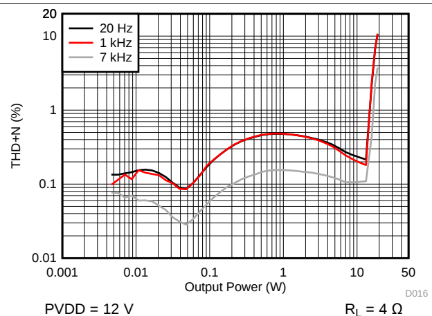
图 20. THD+N vs Output Power - PBTl
