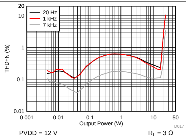
图 21. THD+N vs Output Power - PBTl
