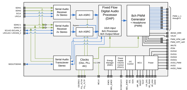
方框图
