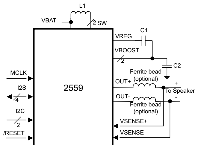
简化原理图
