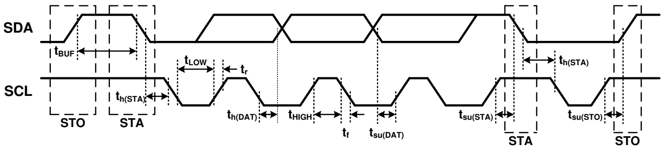
图 1. I²C Timing
