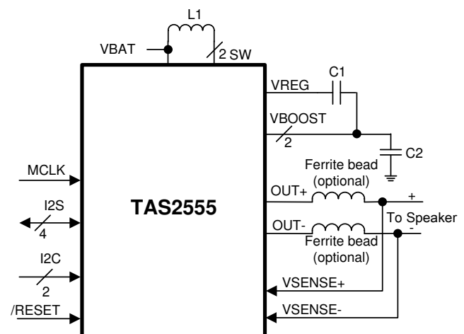
简化原理图
