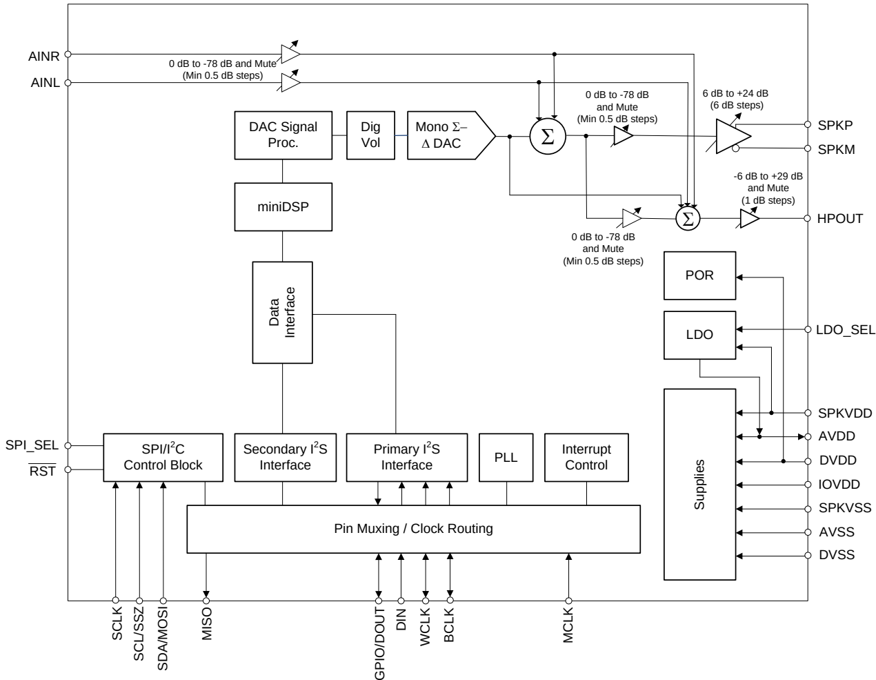
图 1-1. 简化方框图
