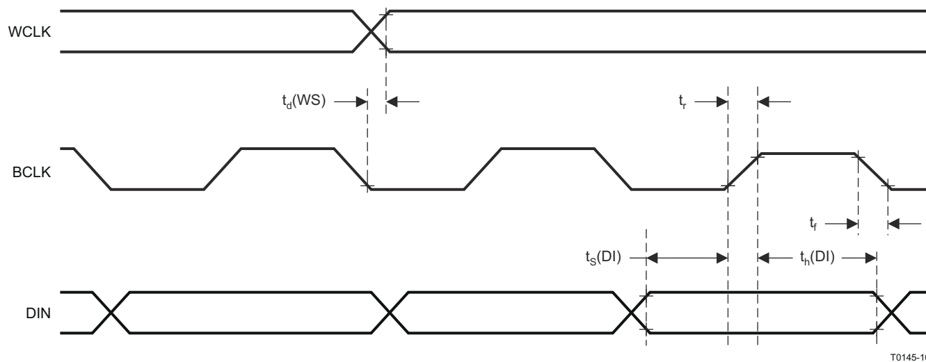
图 5-1. 主模式下的 I²S/LJF/RJF 时序
