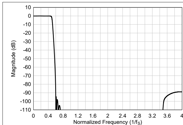
图 6-54. 超低延迟内插滤波器幅度响应
