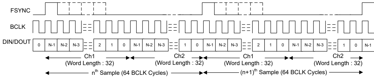
图 6-4. 控制器模式下的 TDM 模式协议时序 ( MD0 短接至 AVDD, 阻值为 4.7K \Omega )
