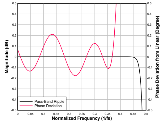
图 6-35. 低延迟内插滤波器通带纹波和相位偏差
