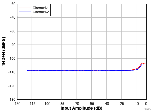
差分输出
