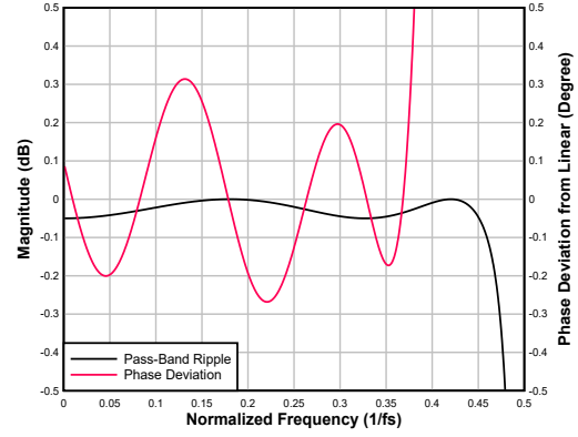
图 6-33. 低延迟内插滤波器通带纹波和相位偏差
