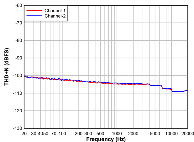
图 5-6. DAC THD+N 级别与频率间的关系
