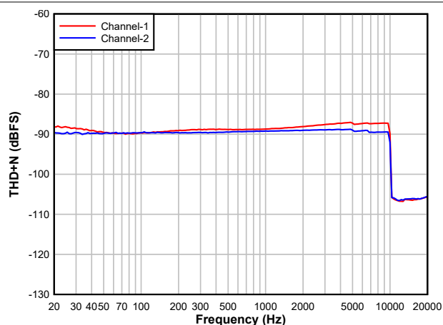
图 5-7. DAC THD+N 级别与频率间的关系
