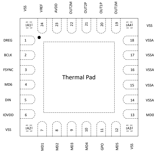
图 4-1. 带有外露散热焊盘和转角引脚的 24 引脚 QFN 封装，顶视图
