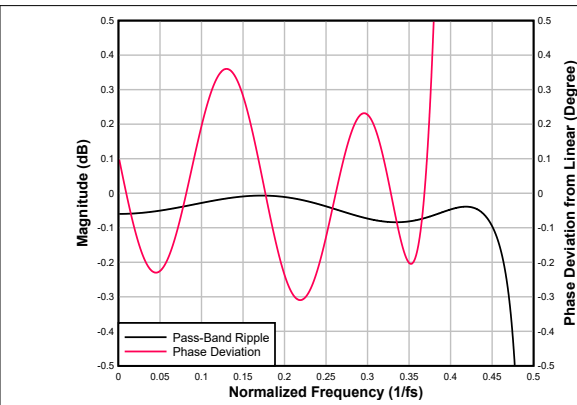
图 6-31. 低延迟内插滤波器通带纹波和相位偏差
