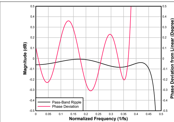
图 6-88. 低延迟内插滤波器通带纹波和相位偏差
