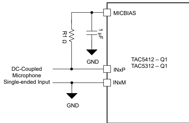
图 6-16. 直流耦合麦克风或线路单端输入连接
