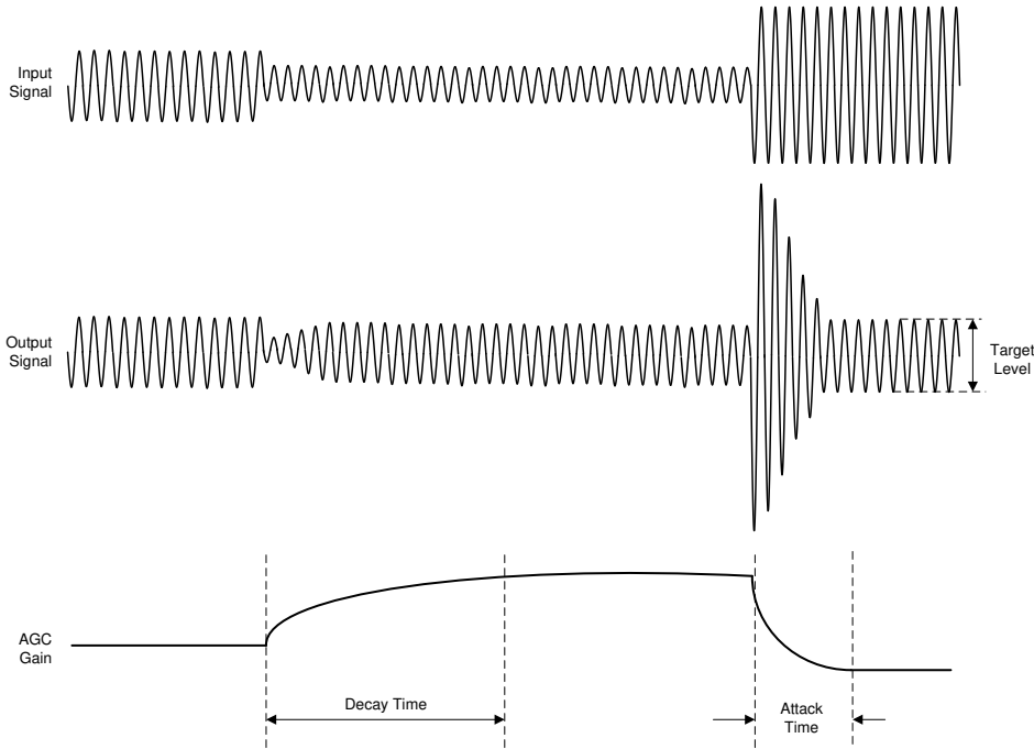
图 6-62. AGC 特性
