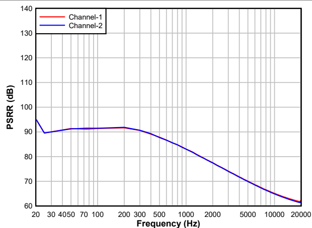
图 5-33. DAC PSRR 与频率间的关系
