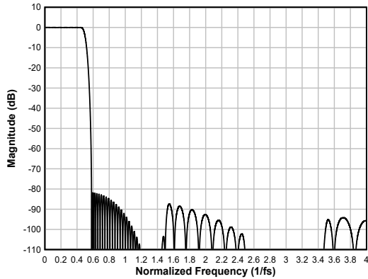
图 6-71. 线性相位内插滤波器幅度响应
