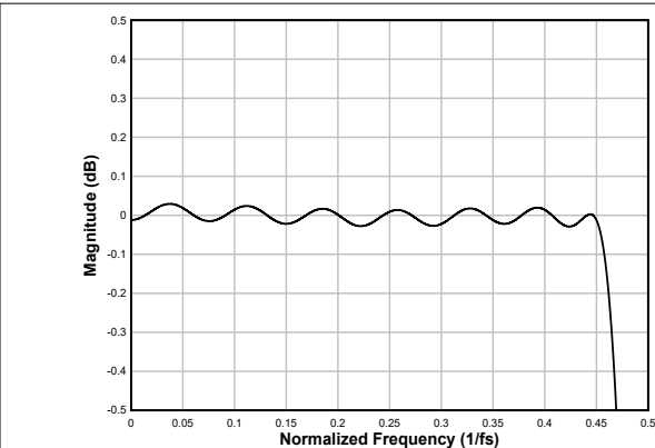
图 6-70. 线性相位内插滤波器通带纹波
