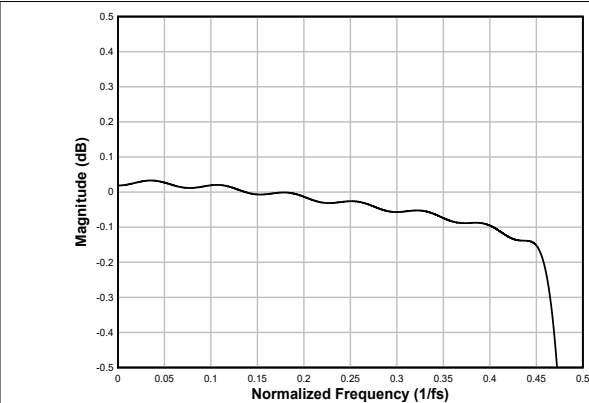
图 6-68. 线性相位内插滤波器通带纹波
