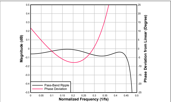
图 6-98. 超低延迟内插滤波器通带纹波和相位偏差
