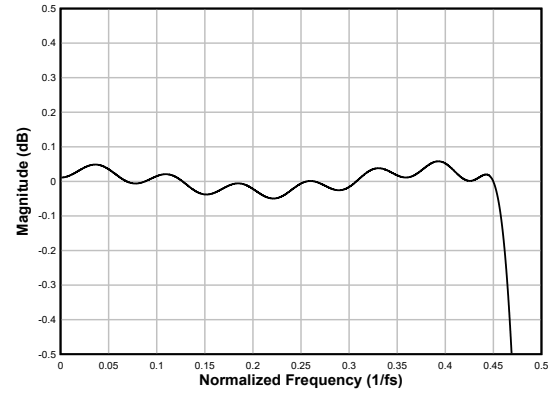
图 6-35. 线性相位抽取滤波器通带纹波
