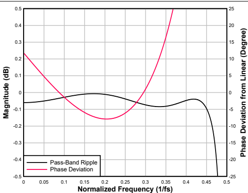
图 7-102. 超低延迟内插滤波器通带纹波和相位偏差
