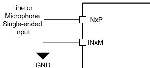
图 7-18. 单端直流耦合输入连接 (ADC_CHx_INSRC 设置为 2'b01、ADC_CHx_CM_TOL 设置为 2'b01 或 2'10)
