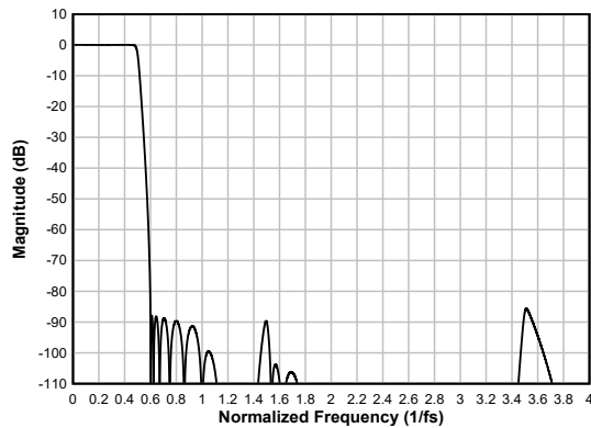
图 7-64. 超低延迟抽取滤波器幅度响应
