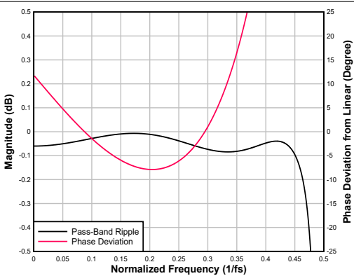
图 7-100. 超低延迟内插滤波器通带纹波和相位偏差
