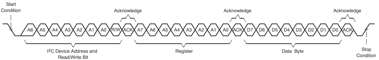
图 7-110. I²C 单字节写入传输
