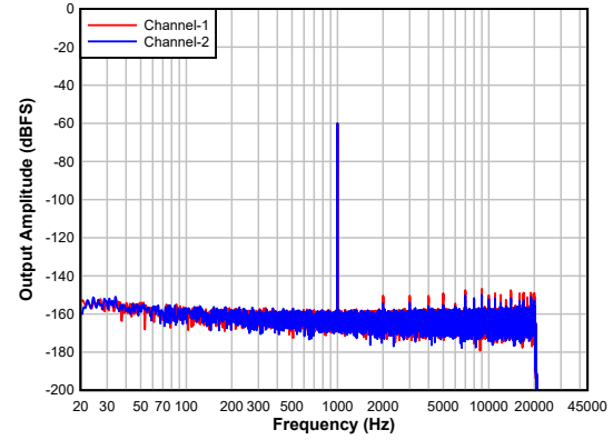
图 6-30. 具有-60dBFS 输入的 DAC FFT
