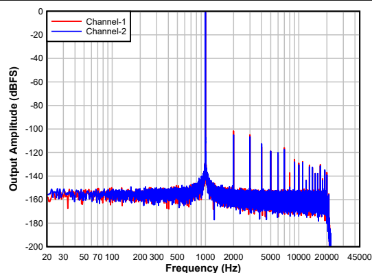
图 6-16. 具有 -1dBFS 输入的 ADC FFT
