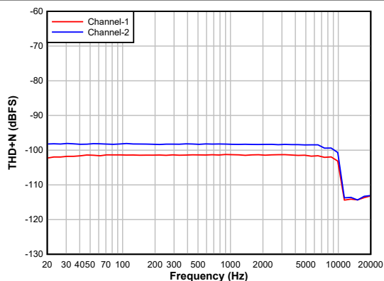
图 6-11. ADC THD+N 与频率间的关系
