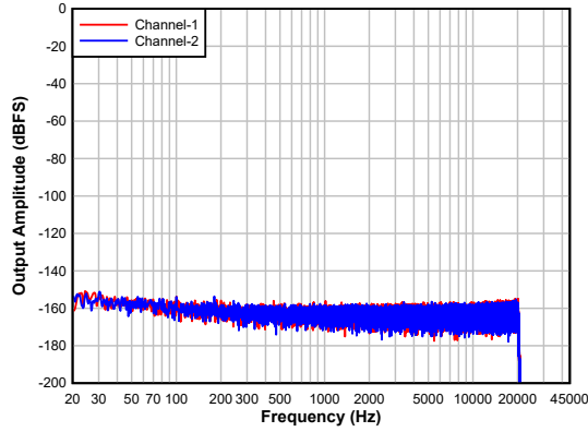
图 6-29. 具有空闲通道输入的 DAC FFT
