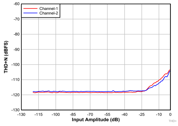
差分输出
