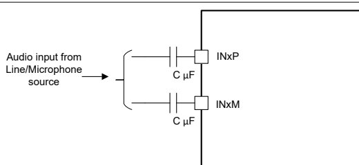
图 7-15. 差分交流耦合输入连接 (ADC_CHx_INSRC 设置为 2'b00、ADC_CHx_CM_TOL 设置为 2'b00 或 2'b01 或 2'10)
