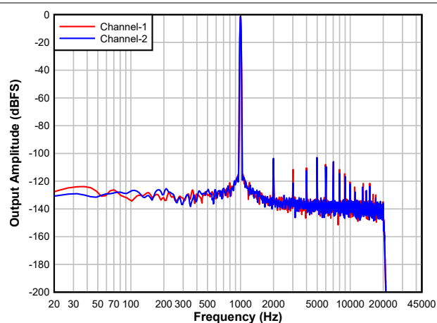
图 6-22. DAC FFT
