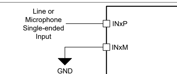
图 7-18. 单端直流耦合输入连接 (ADC_CHx_INSRC 设置为 2'b01、ADC_CHx_CM_TOL 设置为 2'b01 或 2'10)
