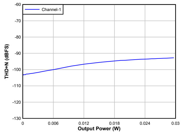
伪差分耳机输出, 16 \Omega 负载
