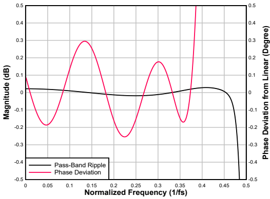
图 6-48. 低延迟抽取滤波器通带纹波和相位偏差
