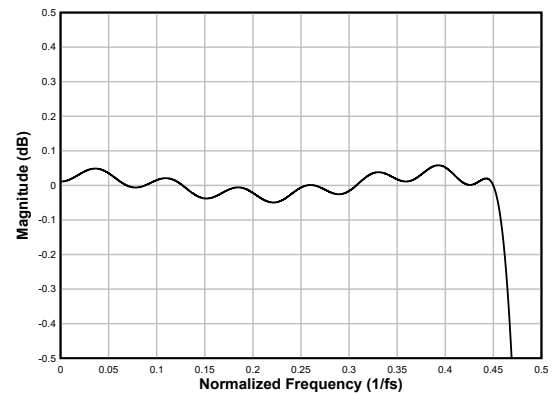
图 6-34. 线性相位抽取滤波器通带纹波
