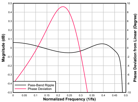
图 6-50. 低延迟抽取滤波器通带纹波和相位偏差
