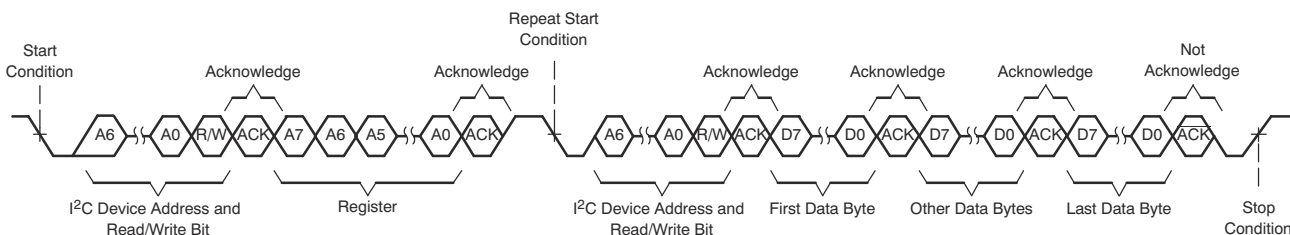
图 6-66. I 2 C 多字节读取传输
