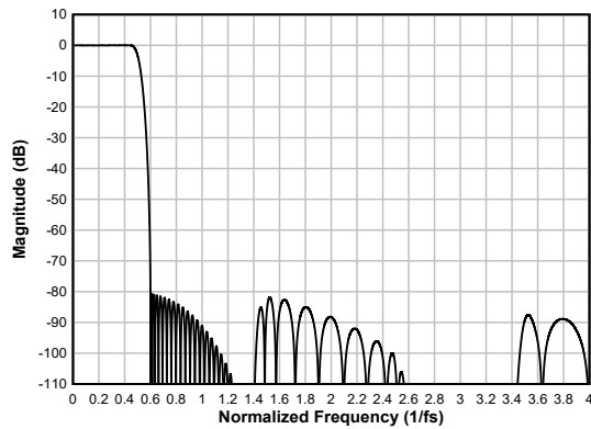
图 6-27. 线性相位抽取滤波器幅度响应
