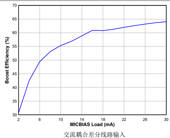
图 5-18. 升压效率与 MICBIAS 负载电流间的关系
