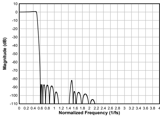
图 6-51. 超低延迟抽取滤波器幅度响应
