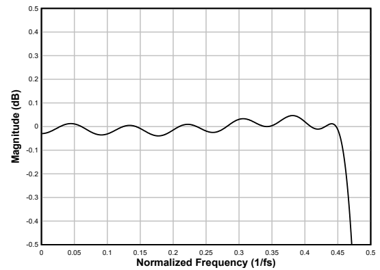
图 6-28. 线性相位抽取滤波器通带纹波
