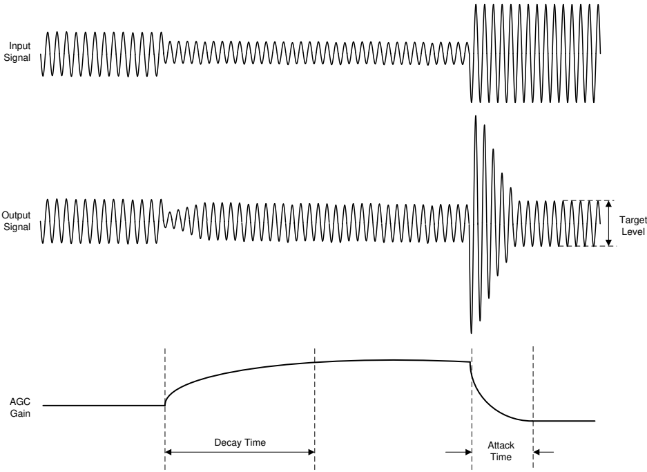
图 6-61. AGC 特性
