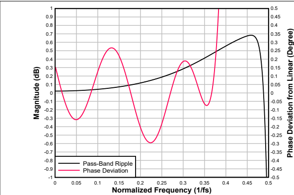
图 6-44. 低延迟抽取滤波器通带纹波和相位偏差
