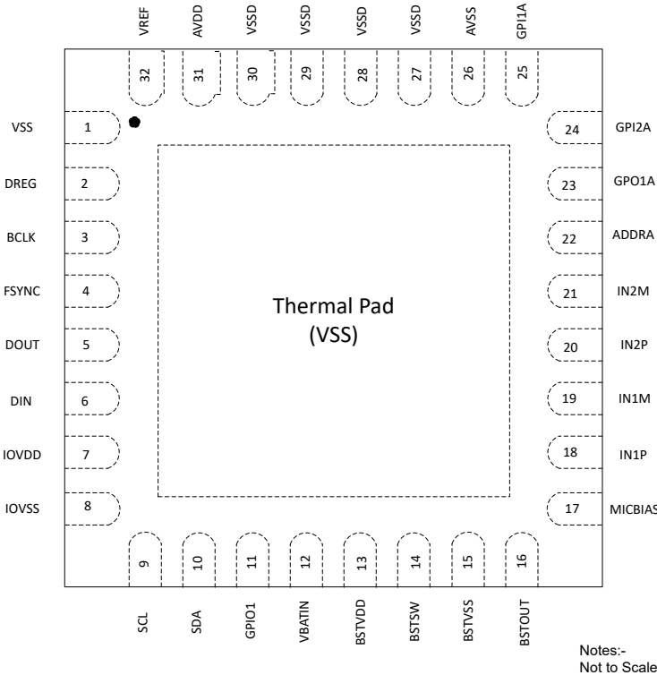
图 4-1. TAA5412-Q1 RTV 封装，32 引脚 WQFN（带有外露散热焊盘），顶视图
