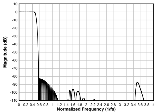
图 6-33. 线性相位抽取滤波器幅度响应
