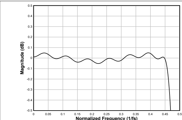
图 6-32. 线性相位抽取滤波器通带纹波
