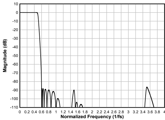
图 6-45. 低延迟抽取滤波器幅度响应
