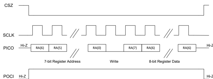
图 6-67. SPI 单字节写入传输
