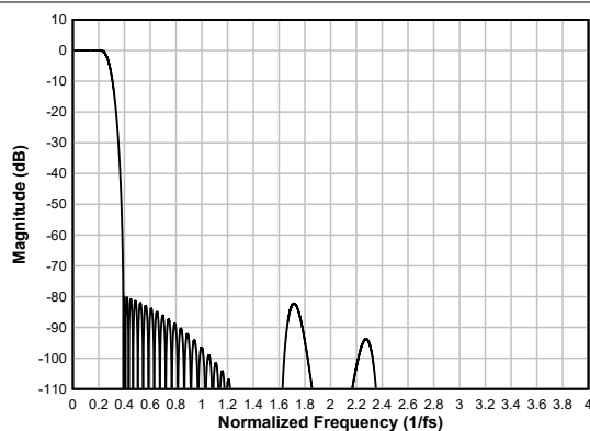
图 6-35. 线性相位抽取滤波器幅度响应
