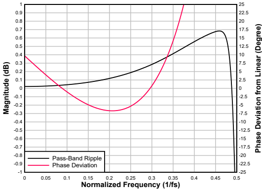
图 6-54. 超低延迟抽取滤波器通带纹波和相位偏差
