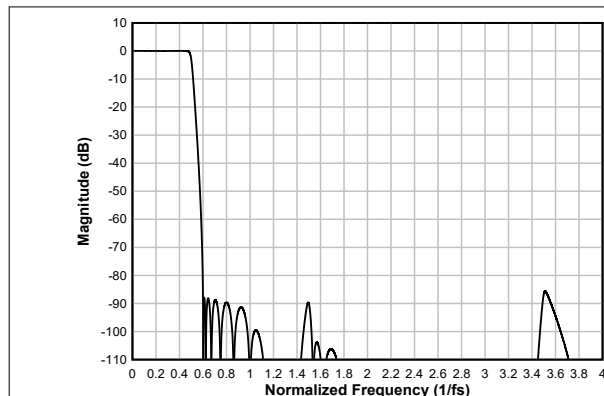
图 6-57. 超低延迟抽取滤波器幅度响应
