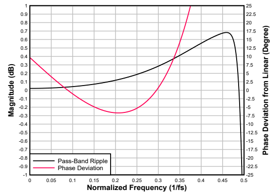
图 6-52. 超低延迟抽取滤波器通带纹波和相位偏差
