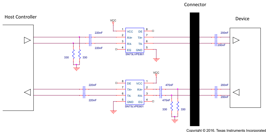
SATA Express 参考原理图
