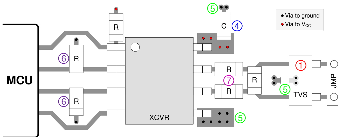
图 12-1. SN65HVD1x Layout Example
