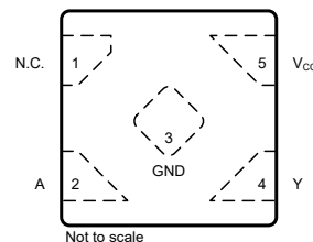
图 4-2. 或 DTX 封装， 5 引脚 X2SON (顶视图)
