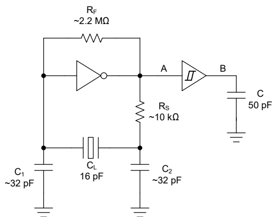
图 8-1. 典型应用原理图
