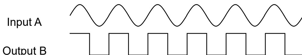
图 8-2. 施密特触发正弦波输入和方波输出
