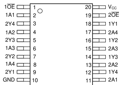
图 4-2. SN74LVCZ244A PW、DW、NS、DB、DGS 封装 (顶视图)
