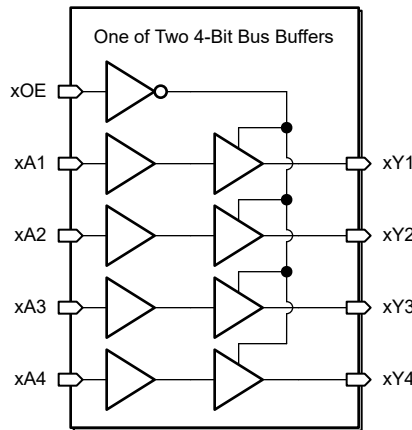
功能方框图
