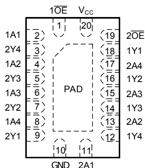
图 4-1. SN74LVCZ244A RKS 封装 (顶视图)
