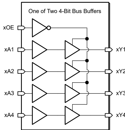
功能方框图
