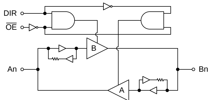
简化原理图
