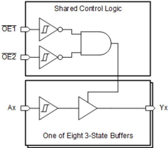
功能方框图
