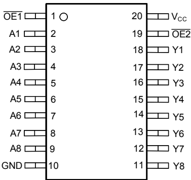
图 4-4. SN74LVC541A PW、DW、NS、DB、 DGS、DGV 封装 (顶视图)
