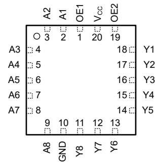
图 4-2. SN54LVC541A FK 封装 (顶视图)
