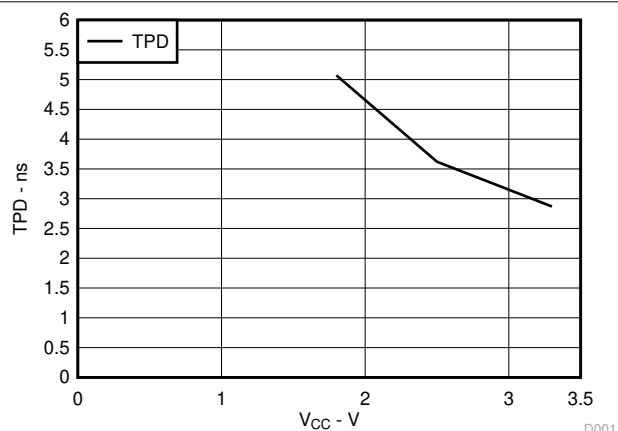
图 5-1. SN74LVC541A 25°C 时 TPD 与 V_{CC} 间的关系
