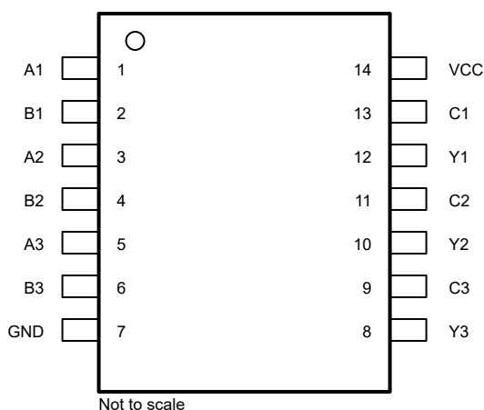
图 4-1. SN74LVC3G97-Q1 PW 封装 ( 预发布 ) , 14 引脚 TSSOP ( 顶视图 )
