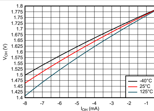
图 5-10. 高电平状态下输出电压与电流间的关系 (1.8V 电源)
