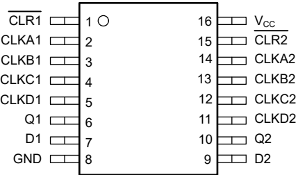
图 4-2. PW 封装，16 引脚 TSSOP（预发布）（顶视图）
