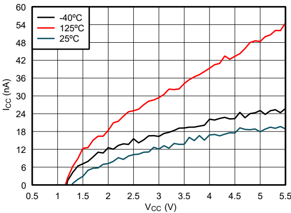
图 5-1. 整个电源电压和温度范围内的电源电流
