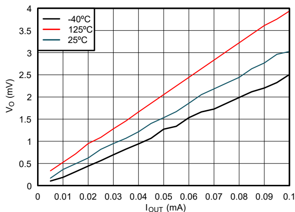
图 5-7. 低电平状态下输出电压与电流间的关系 (1.38V 电源)
