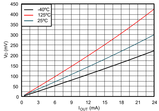
图 5-4. 低电平状态下输出电压与电流间的关系 (3V 电源)
