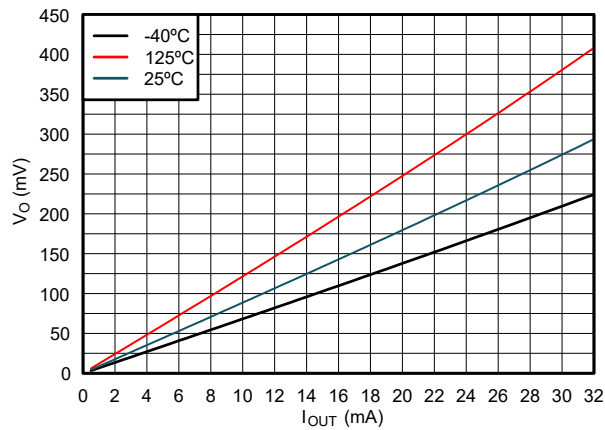
图 5-3. 低电平状态下输出电压与电流间的关系 (4.5V 电源)
