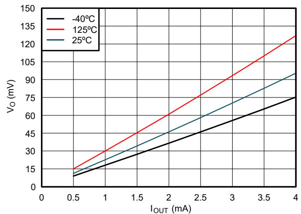
图 5-6. 低电平状态下输出电压与电流间的关系 (1.65V 电源)
