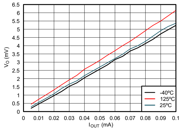
图 5-8. 低电平状态下输出电压与电流间的关系 (1.1V 电源)
