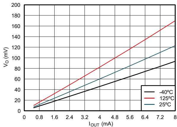
图 5-5. 低电平状态下输出电压与电流间的关系 (2.3V 电源)
