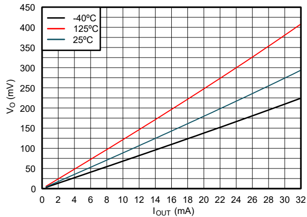
图 5-4. 低电平状态下输出电压与电流间的关系 (4.5V 电源)
