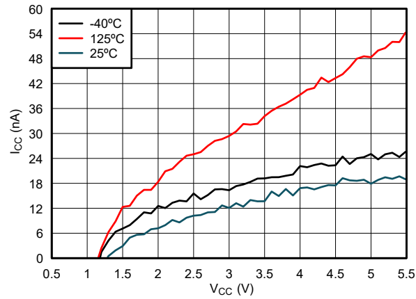
图 5-1. 整个电源电压和温度范围内的电源电流
