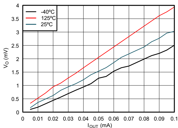
图 5-8. 低电平状态下输出电压与电流间的关系 ( 1.38V 电源 )
