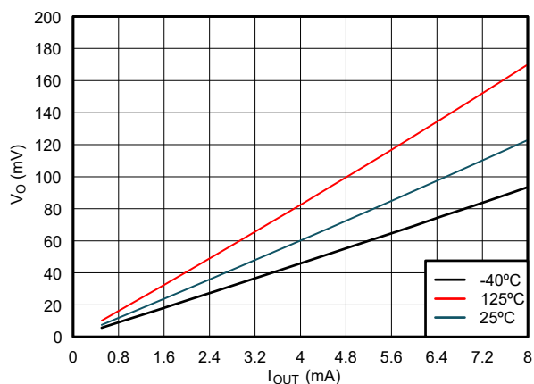
图 5-6. 低电平状态下输出电压与电流间的关系 ( 2.3V 电源 )
