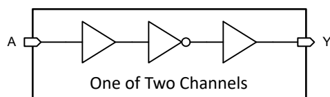
图 7-1. 逻辑图 (正逻辑)
