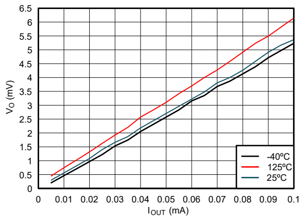
图 5-9. 低电平状态下输出电压与电流间的关系 ( 1.1V 电源 )
