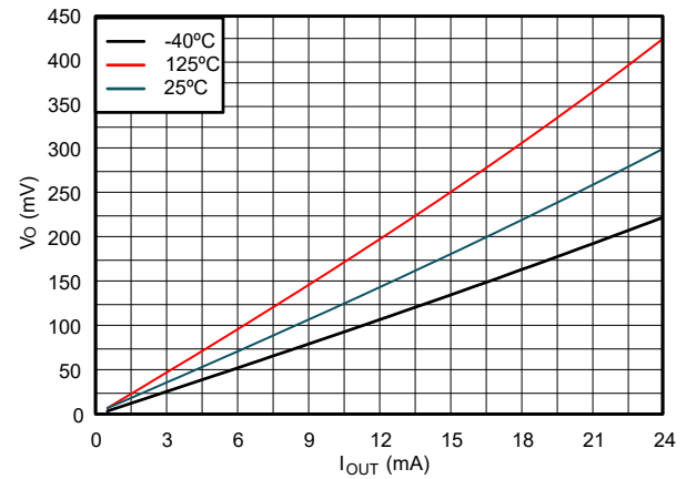
图 5-5. 低电平状态下输出电压与电流间的关系 (3V 电源)
