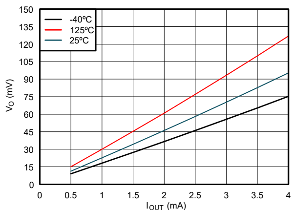
图 5-7. 低电平状态下输出电压与电流间的关系 ( 1.65V 电源 )
