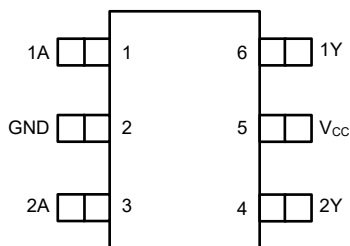
图 4-1. DBV, DCK 封装, 6 引脚 SOT-23, SOT-SC70 (顶视图)
