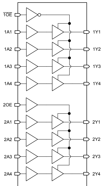
图 7-1. 逻辑图 (正逻辑)
