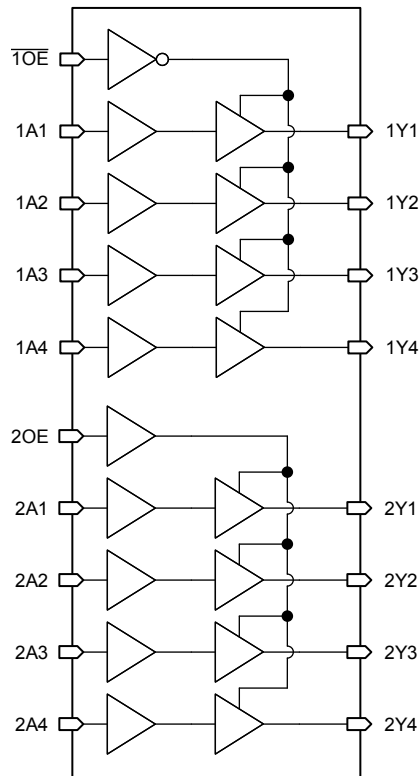
功能方框图
