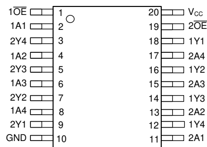
图 4-2. SN74LVC240A-Q1 PW、DGS 封装 (顶视图)
