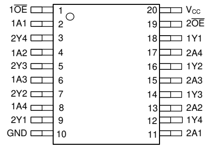
图 4-2. SN74LVC240A PW、DW、NS、DB、DGS、DGV 封装 (顶视图)
